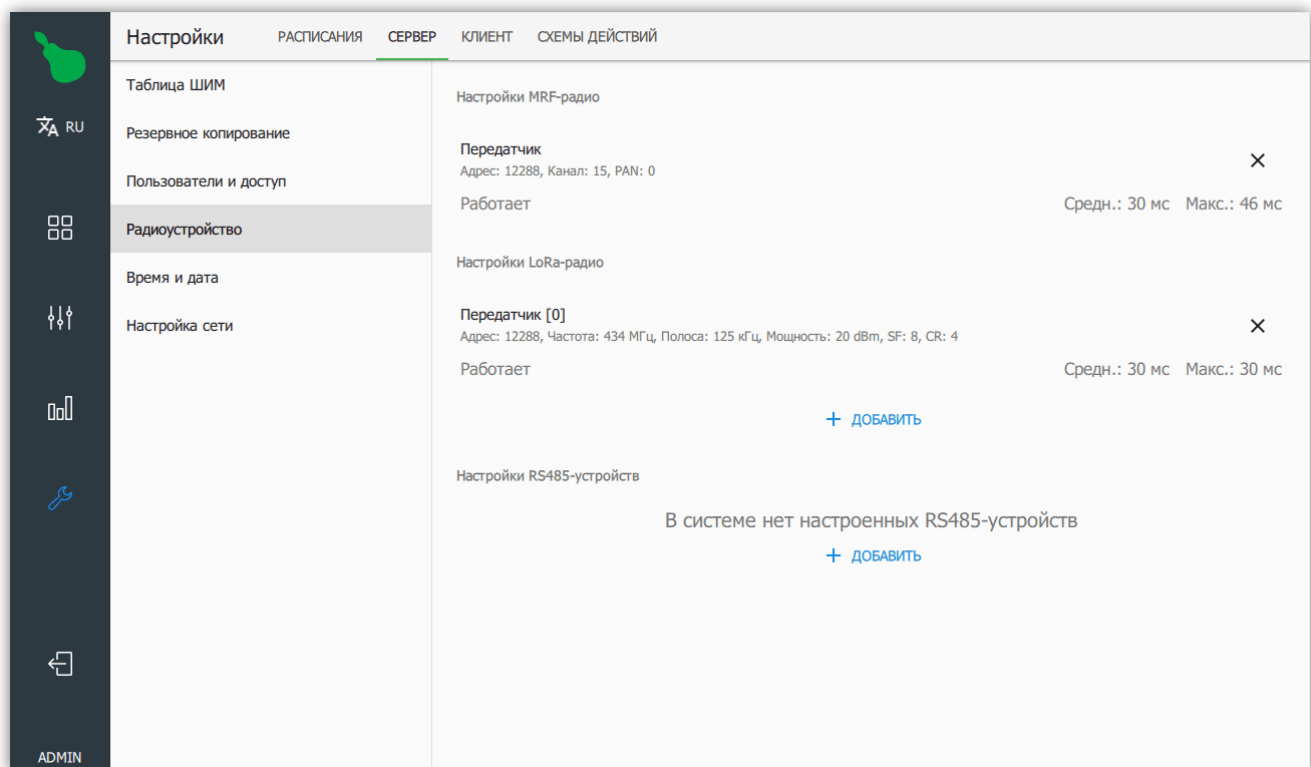
Рисунок 53. Настройка радиоустройств
