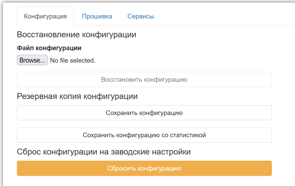
Рисунок 78. Вкладка конфигурации
