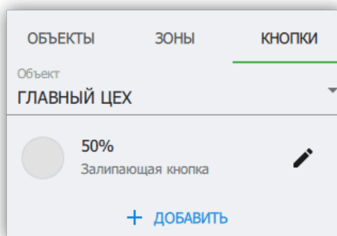
Рисунок 25. Список кнопок
