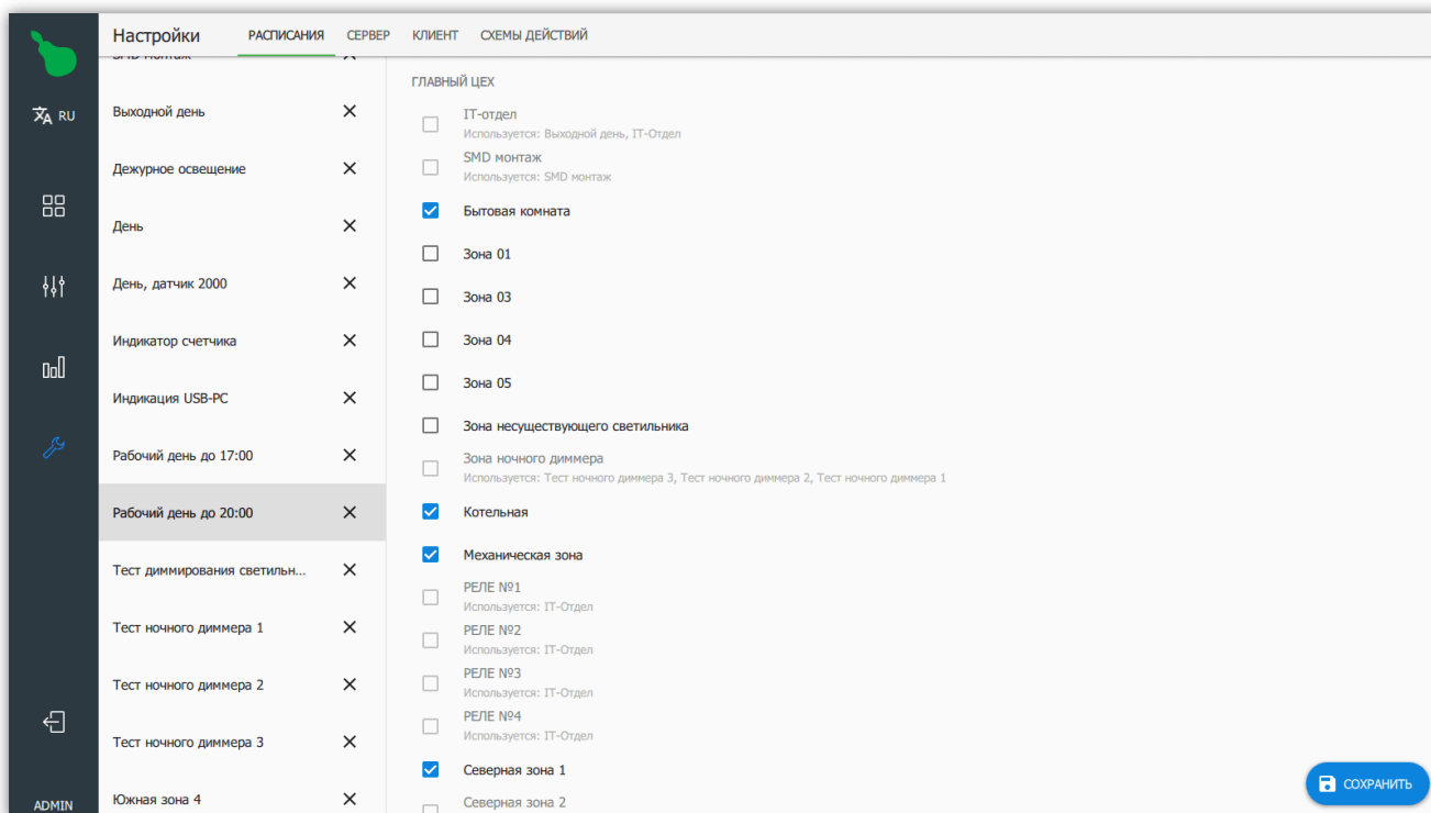
Рисунок 48. Зоны расписания
