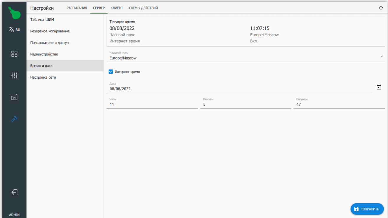
Рисунок 56. Настройки времени
