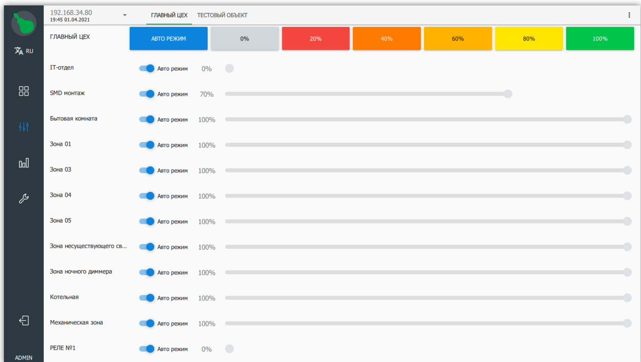
Рисунок 35. Вкладка управления
