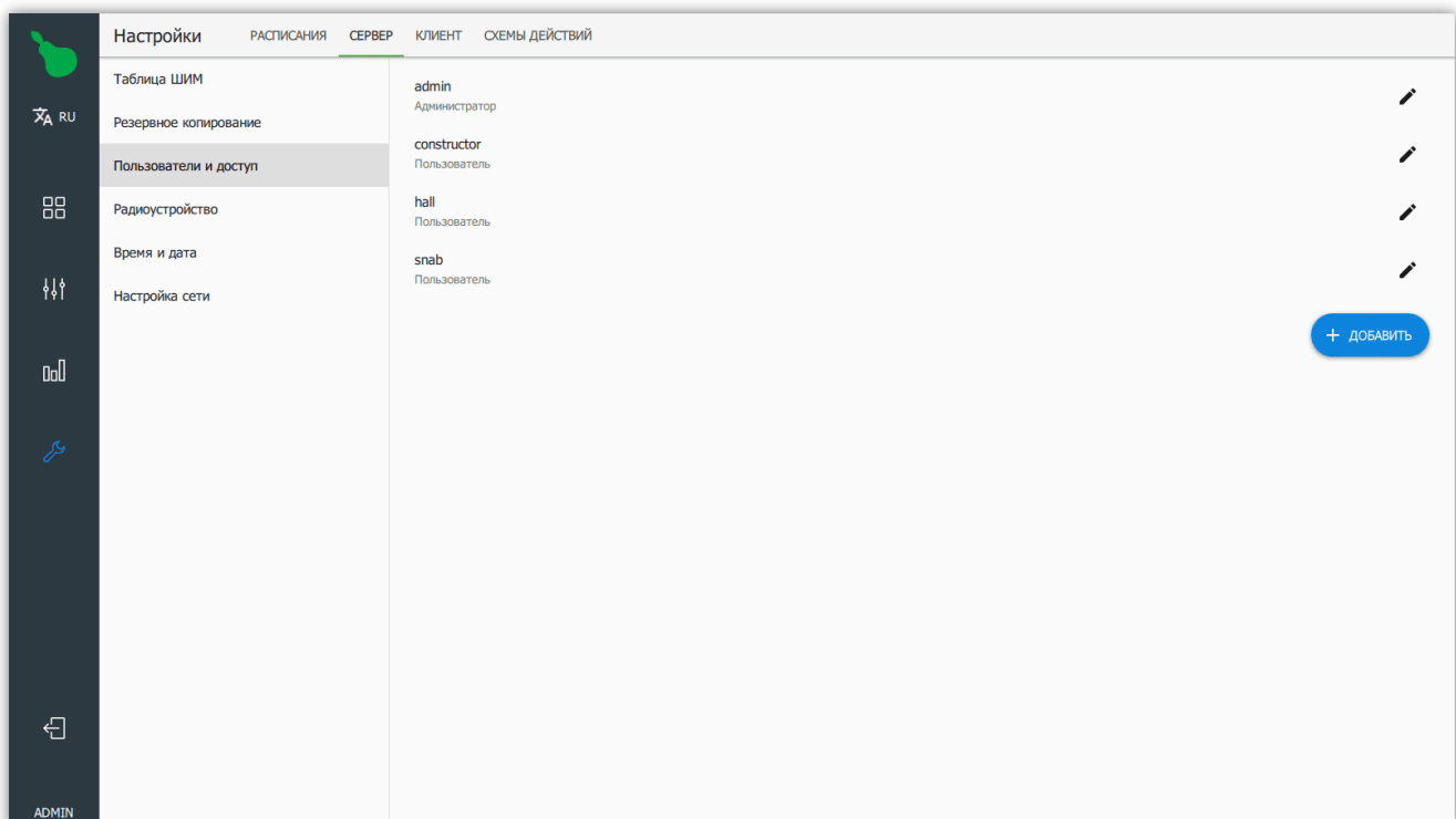
Рисунок 51. Список пользователей
