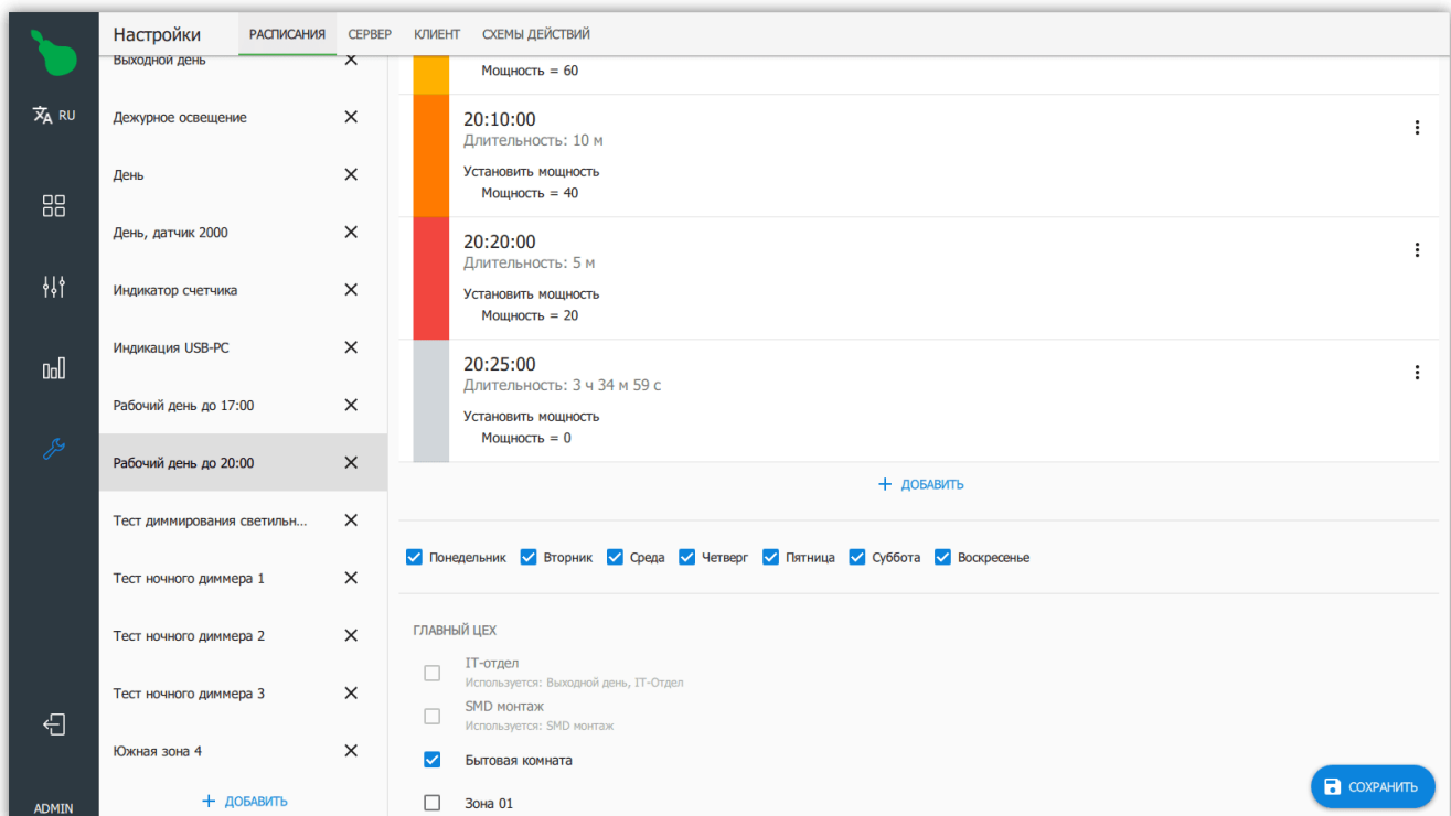
Рисунок 45. Редактирование расписаний
