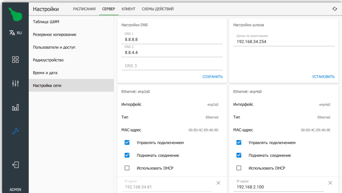
Рисунок 57. Настройка сети
