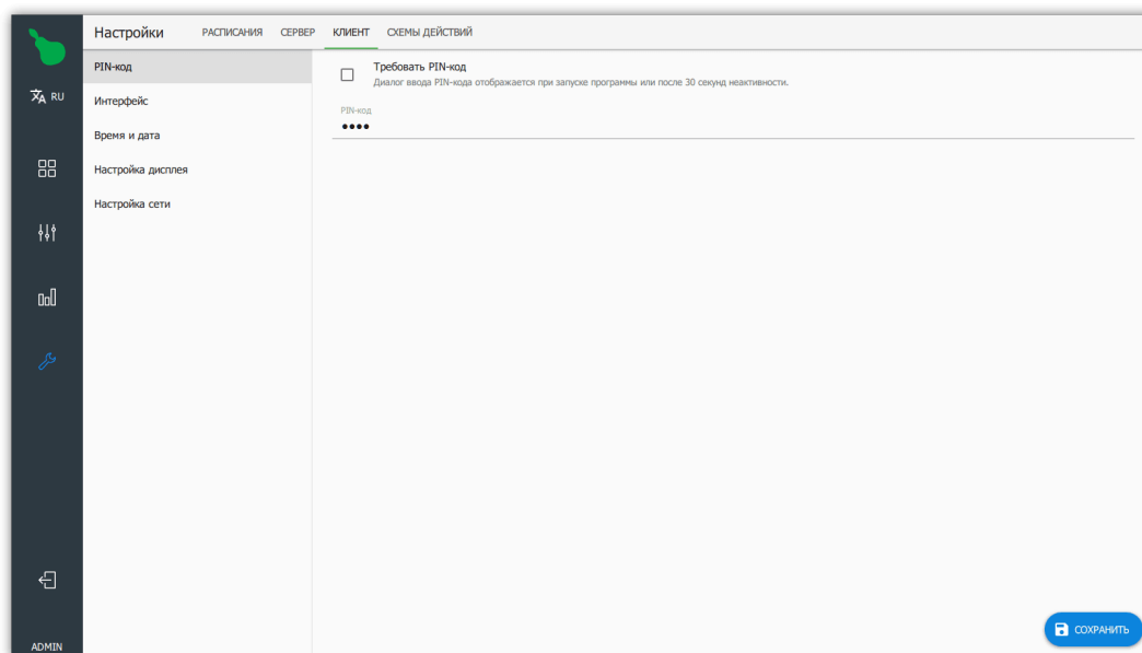
Рисунок 60. Настройки PIN-кода
