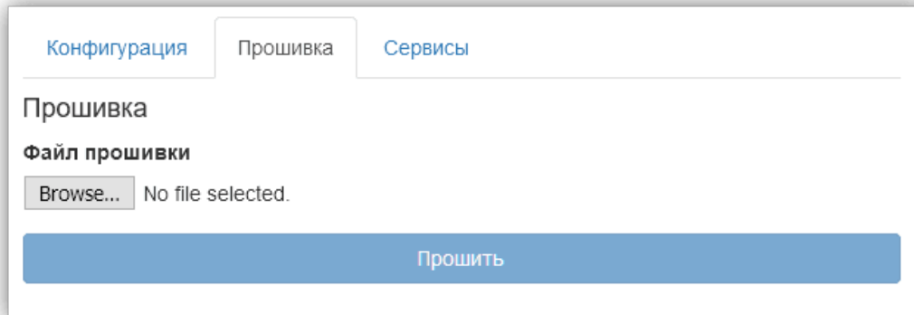
Рисунок 79. Вкладка "Прошивка"
