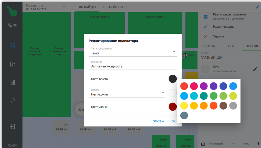
Рисунок 31. Редактирование индикатора
