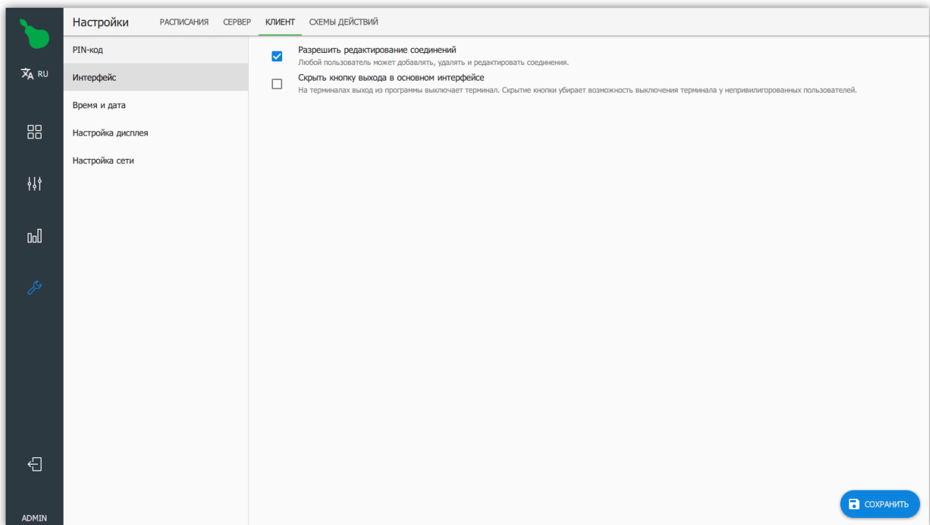
Рисунок 62. Настройки интерфейса
