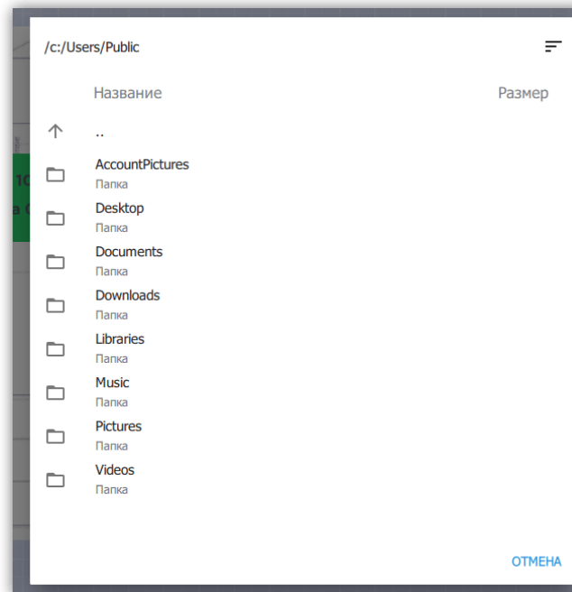
Рисунок 32. Файловый диалог
