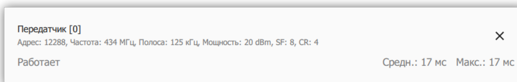
Рисунок 51. Информация о LoRa-передатчике
