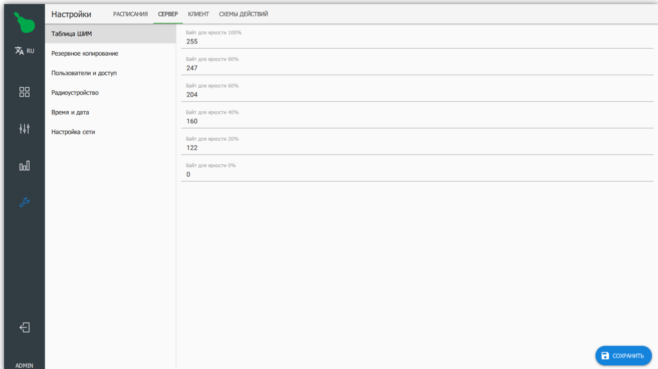
Рисунок 45. Настроенная таблица ШИМ для блоков питания Mean Well
