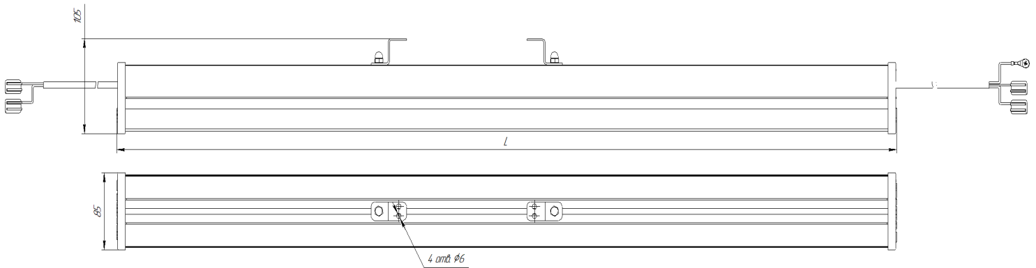
Рисунок 1. Габаритный чертёж Econex Loft
