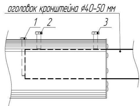
Рисунок 8. Установка светильника Econex Road
