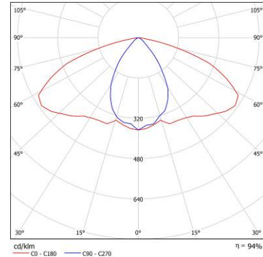
Рисунок 5. КСС типа Ш3 (Широкая осевая)
