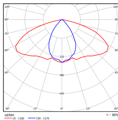
Рисунок 2. КСС типа ШЗ (широкая)
