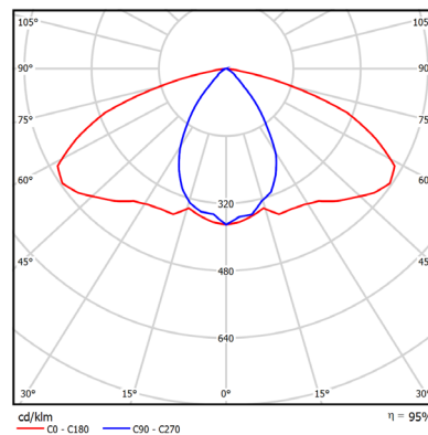
Рисунок 2. КСС типа ШЗ (широкая)
