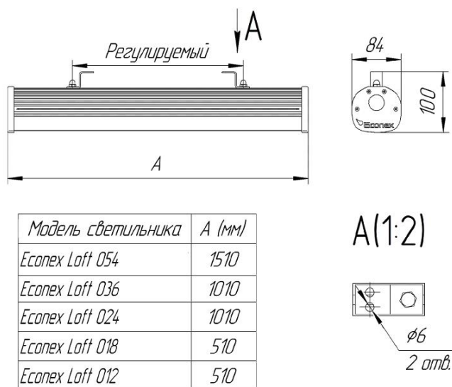
Рисунок 1. Габаритный чертеж Econex Loft
