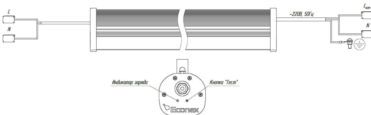
Рисунок 4. Подключение светодиодного светильника Econex Loft EM
