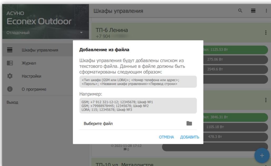
Рисунок 18. Массовое добавление из файла
