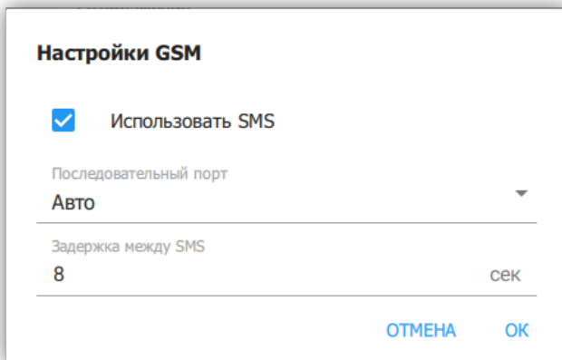
Рисунок 29. Диалог настроек GSM
