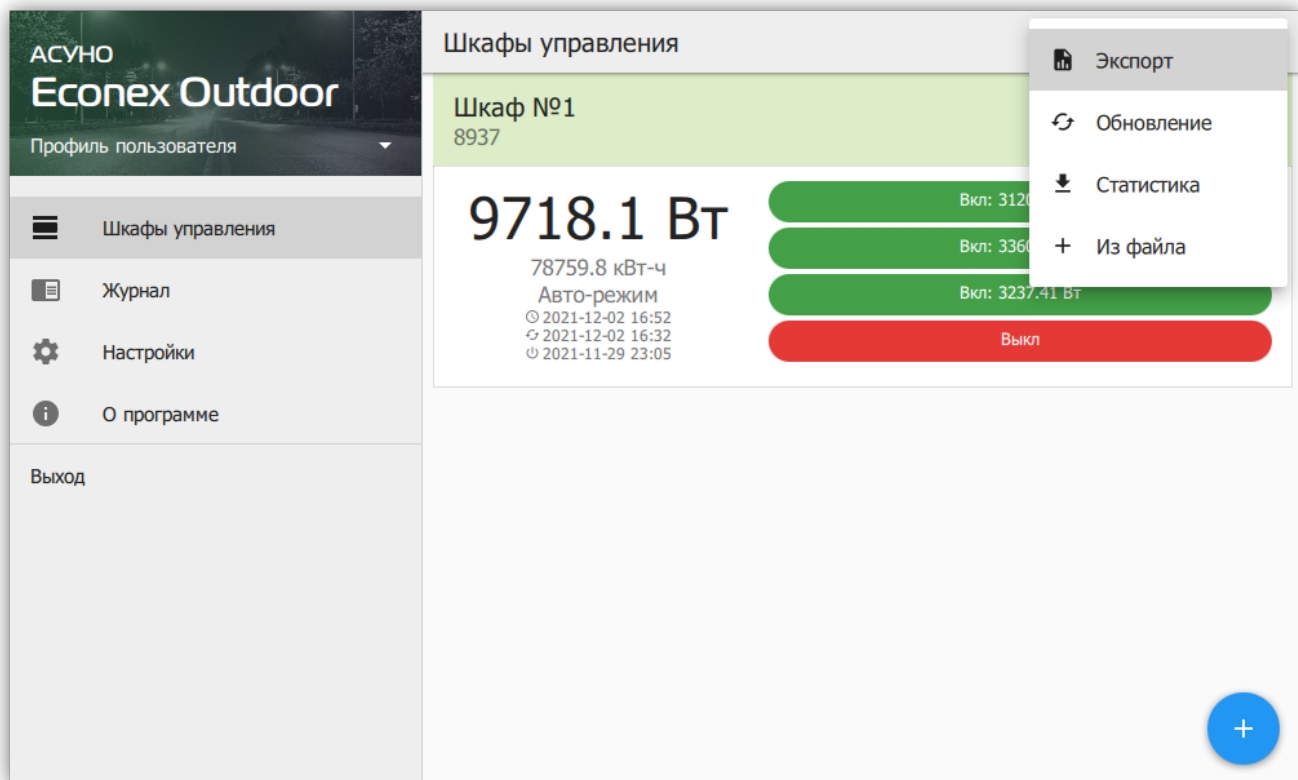
Рисунок 16. Меню действий
