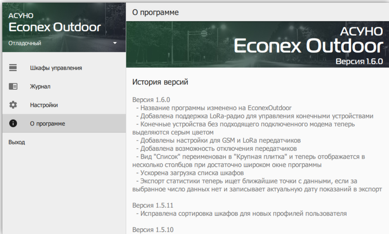
Рисунок 32. О программе
