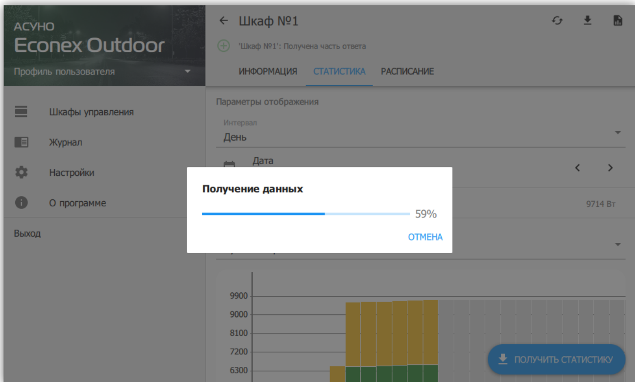
Рисунок 22. Загрузка статистики
