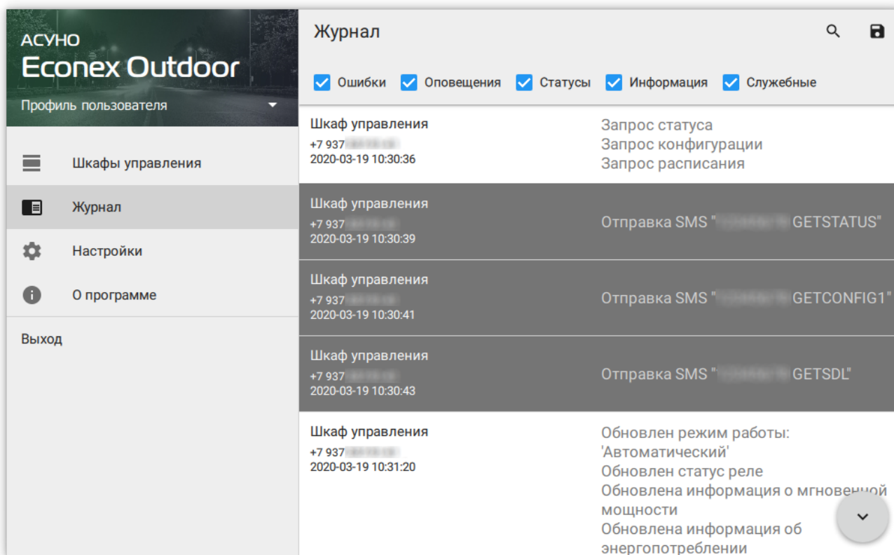
Рисунок 28. Журнал
