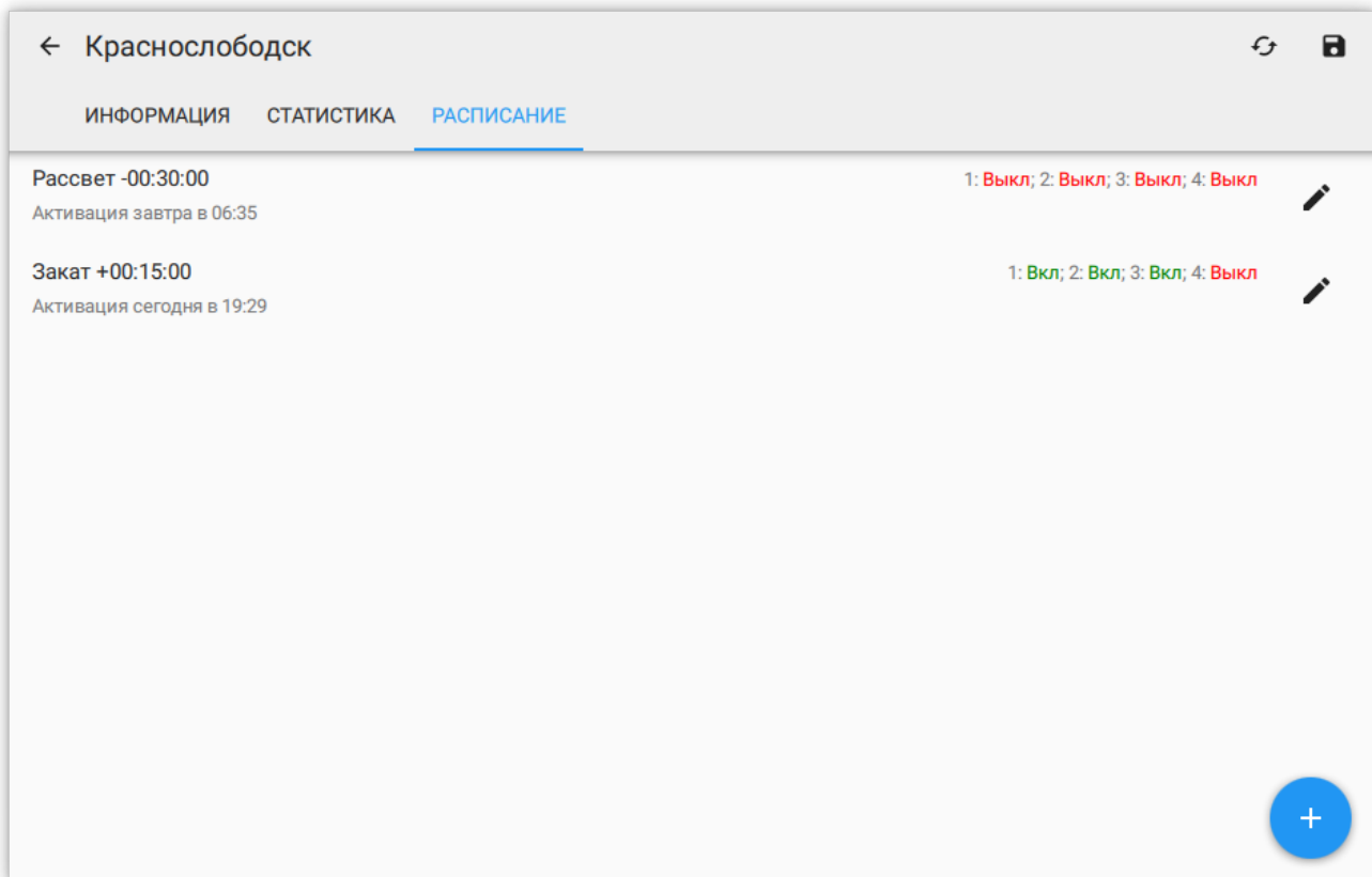
Рисунок 26. Список расписаний
