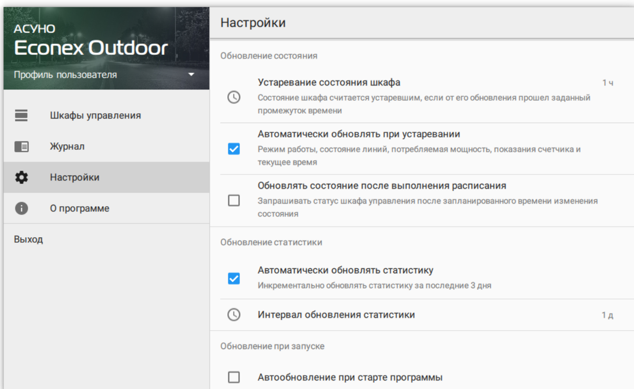
Рисунок 31. Настройки
