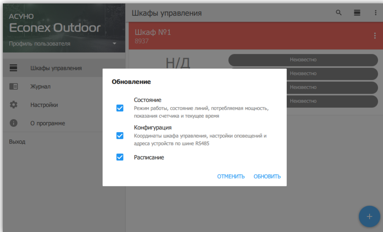
Рисунок 5. Диалог обновления
