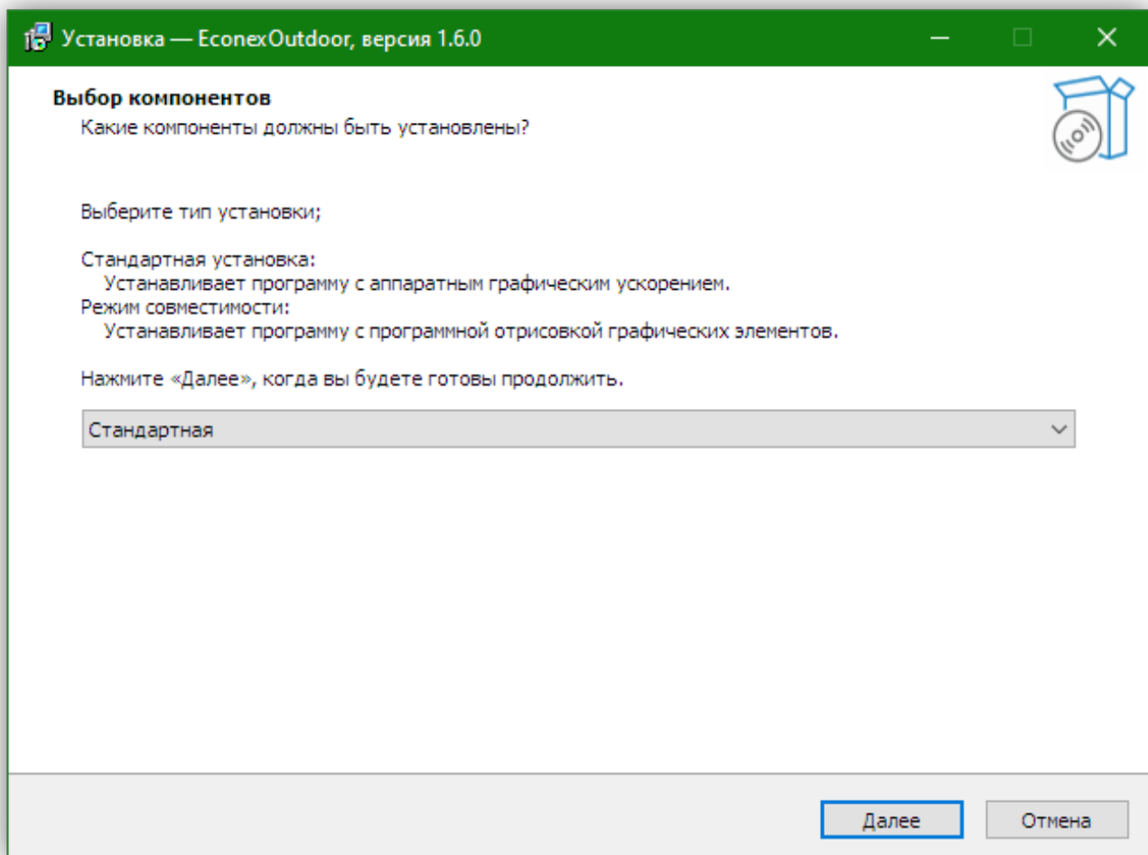
Рисунок 1. Мастер установки
