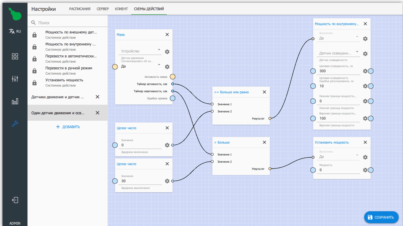
Рисунок 66. Схема действия
