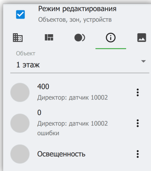
Рисунок 26. Список индикаторов
