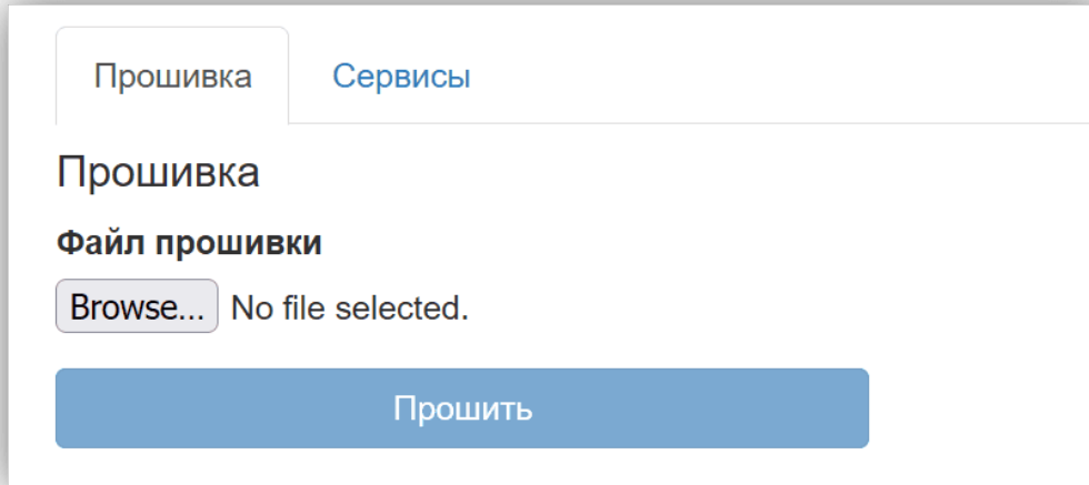
Рисунок 82. Вкладка "Прошивка"
