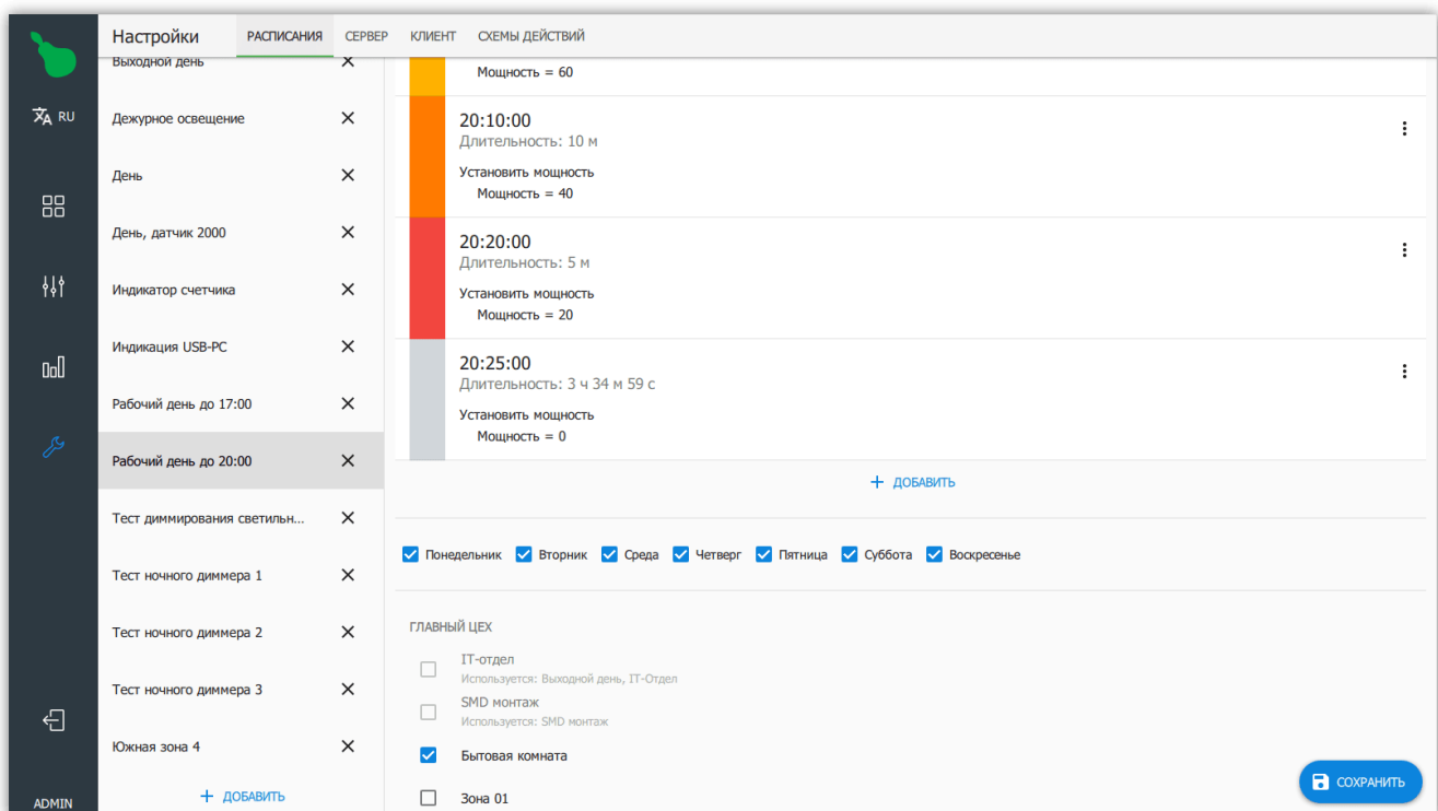
Рисунок 47. Редактирование расписаний
