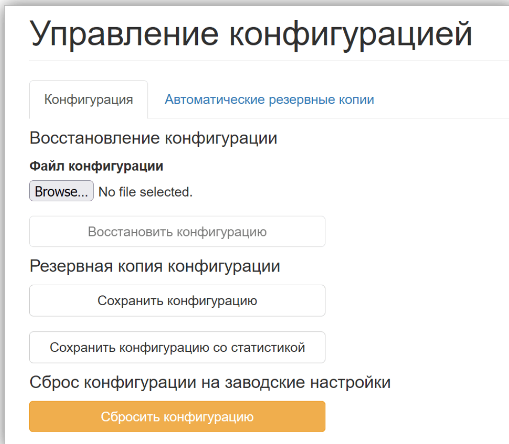
Рисунок 79. Вкладка конфигурации
