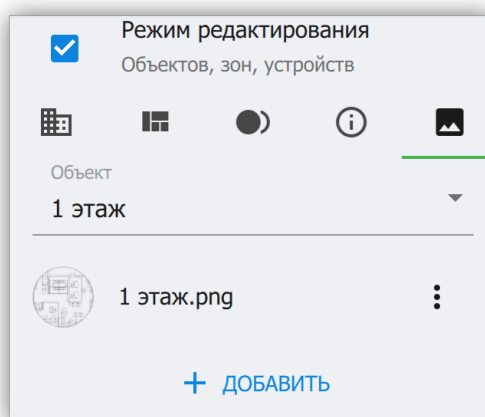
Рисунок 27. Список изображений
