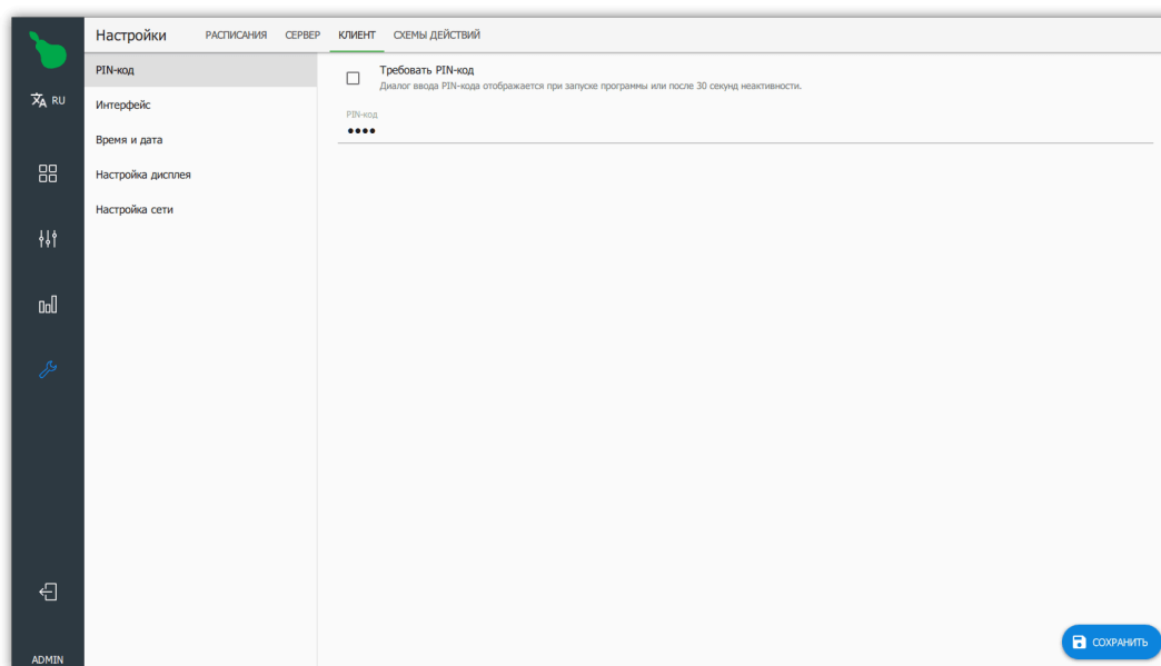
Рисунок 62. Настройки PIN-кода
