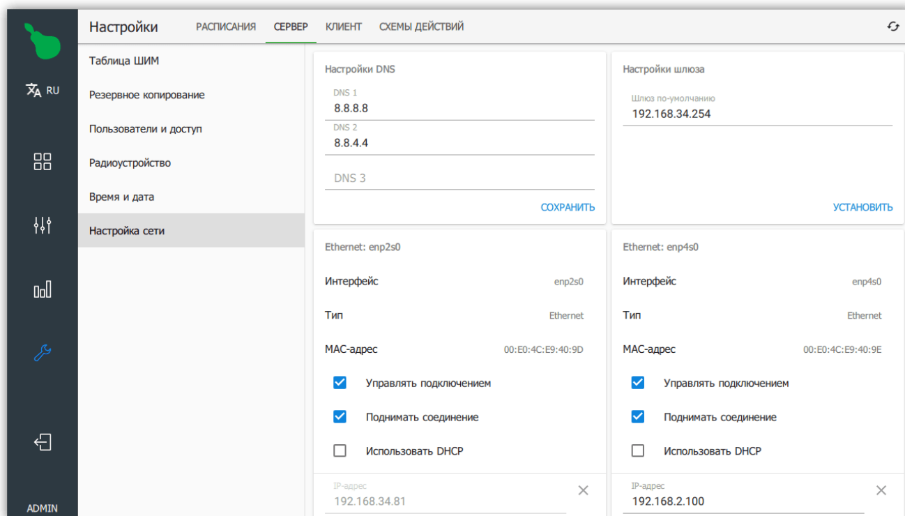
Рисунок 59. Настройка сети
