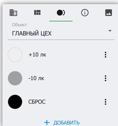
Рисунок 25. Список кнопок
