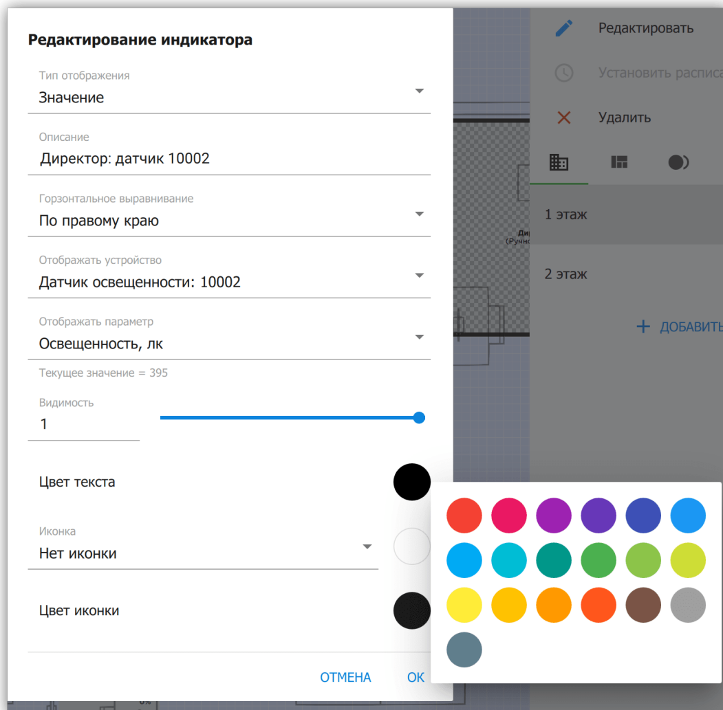
Рисунок 33. Редактирование индикатора
