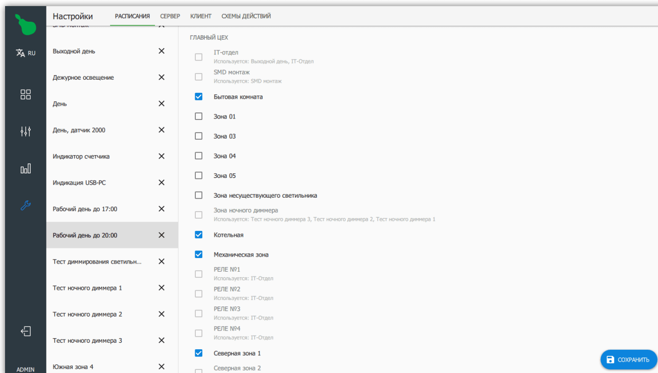
Рисунок 50. Зоны расписания
