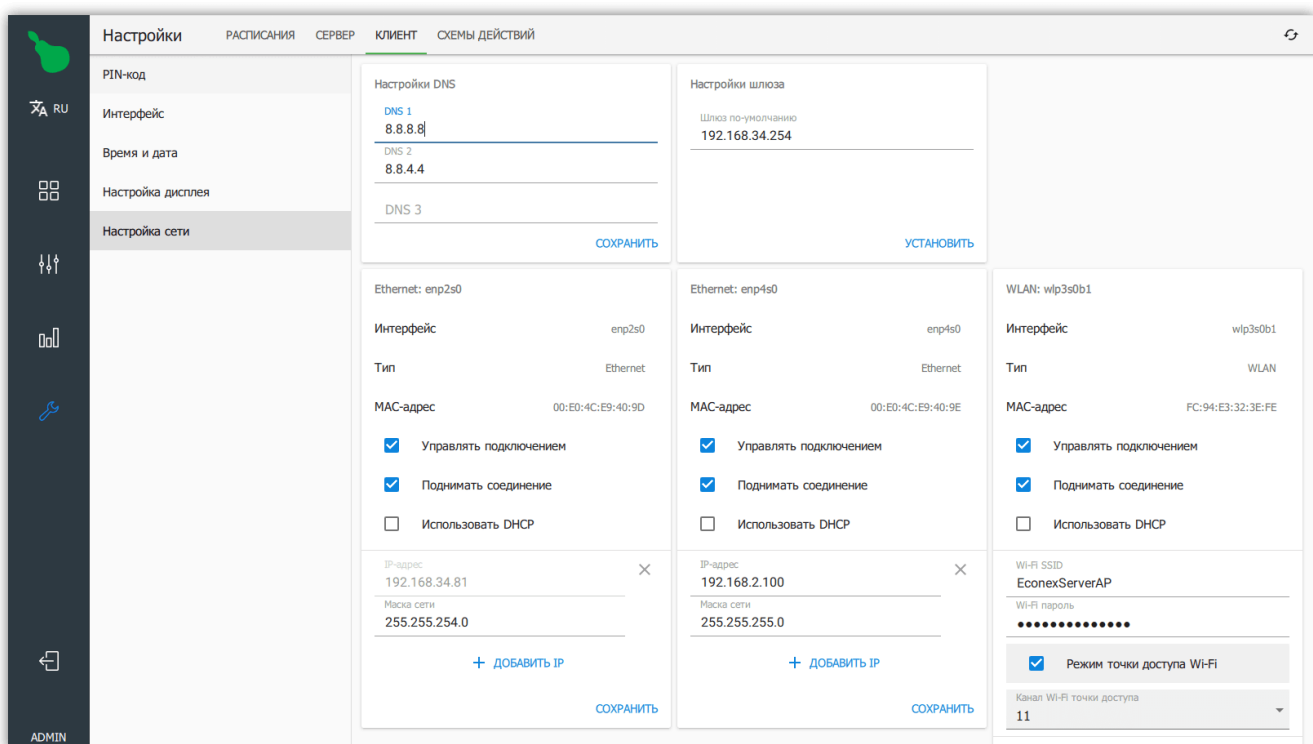
Рисунок 65. Настройки сети
