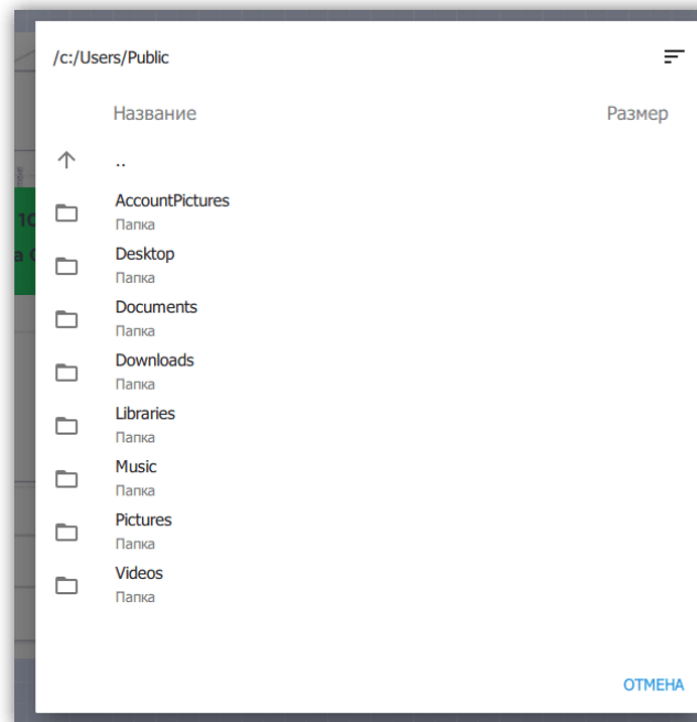
Рисунок 34. Файловый диалог
