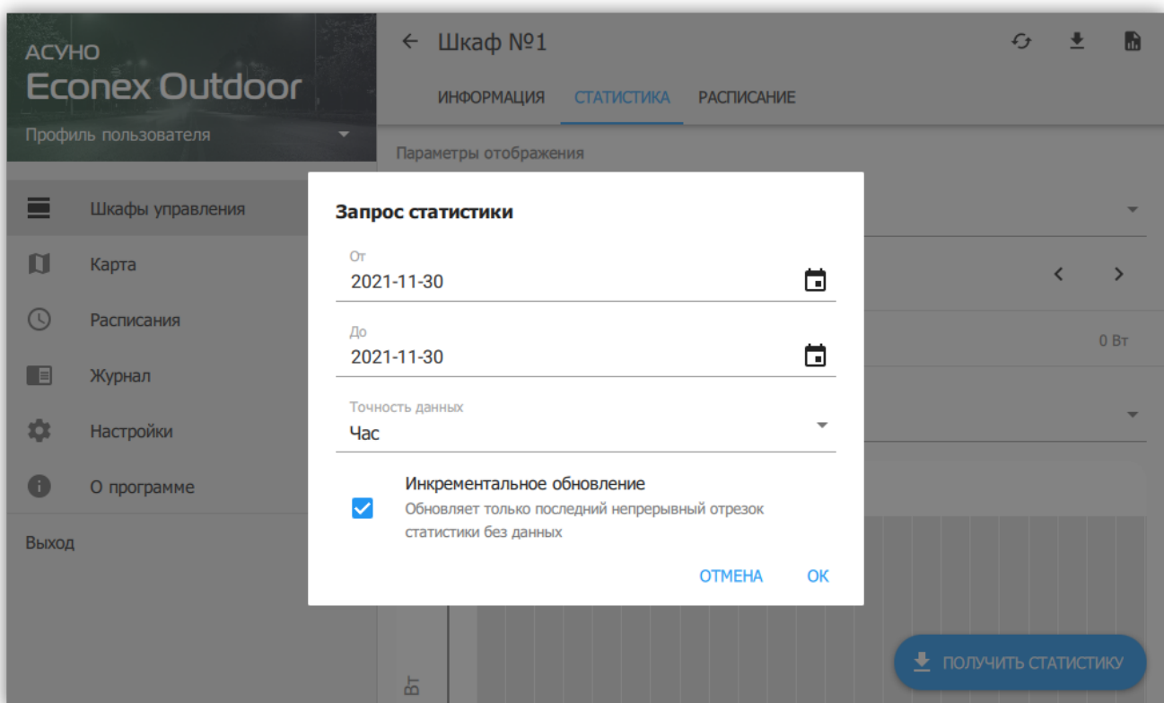
Рисунок 20. Диалог загрузки статистики
