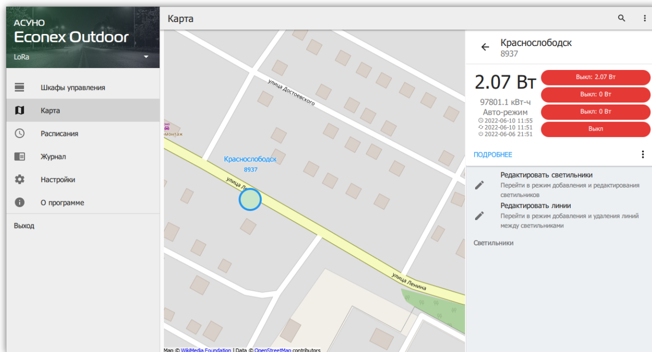
Рисунок 27. Отображение на карте
