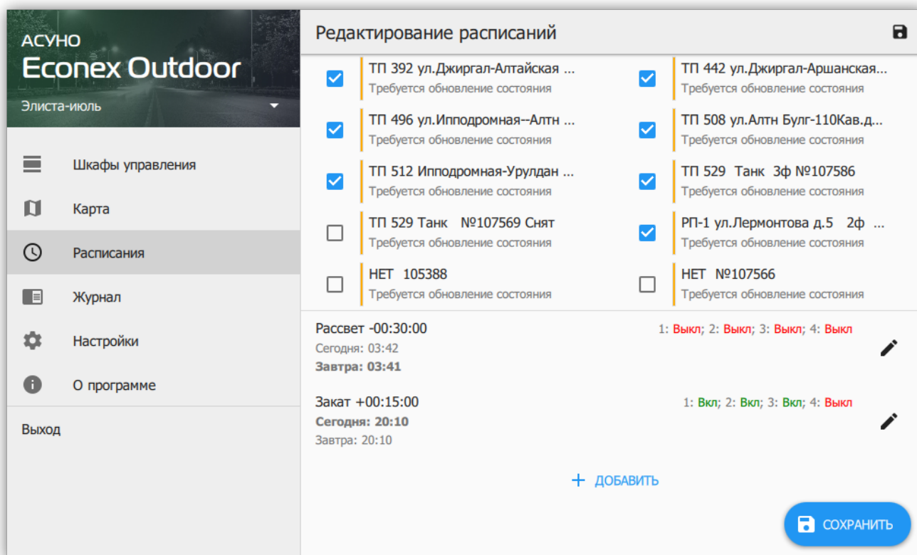
Рисунок 30. Редактирование расписаний нескольких шкафов
