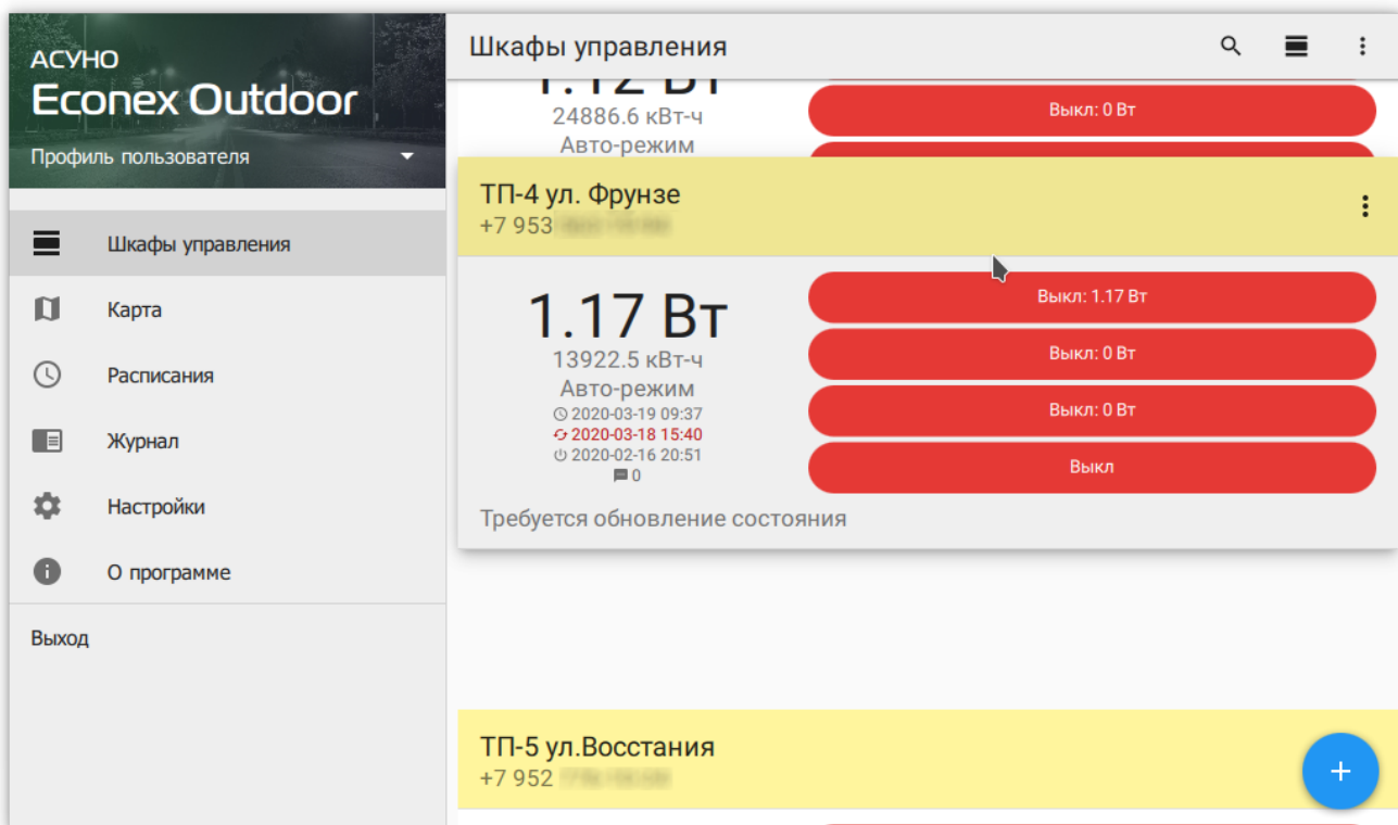
Рисунок 10. Изменение порядка устройств в списке
