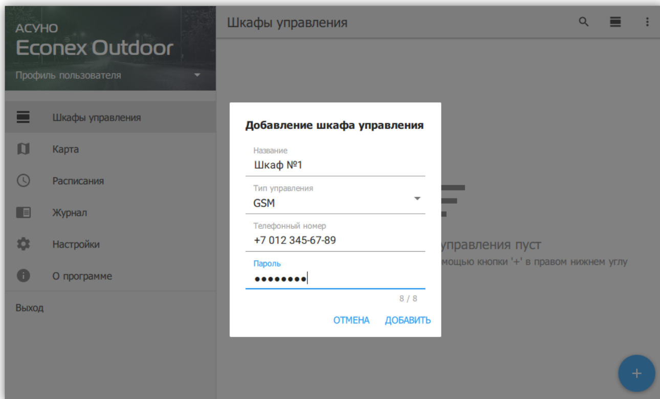
Рисунок 14. Диалог добавления устройства
