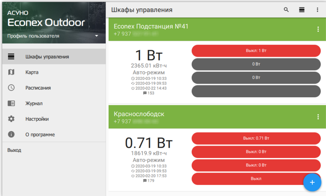
Рисунок 11. Крупная плитка при малом размере окна
