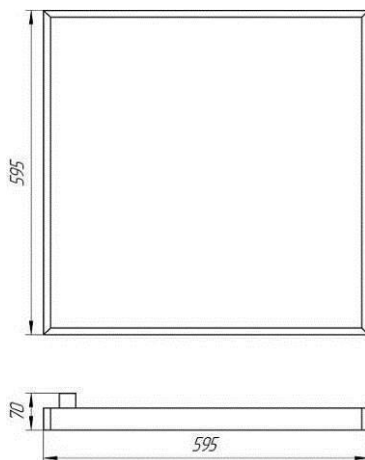
Рисунок 1. Габаритный чертеж Econex Office EM (встраиваемый)
