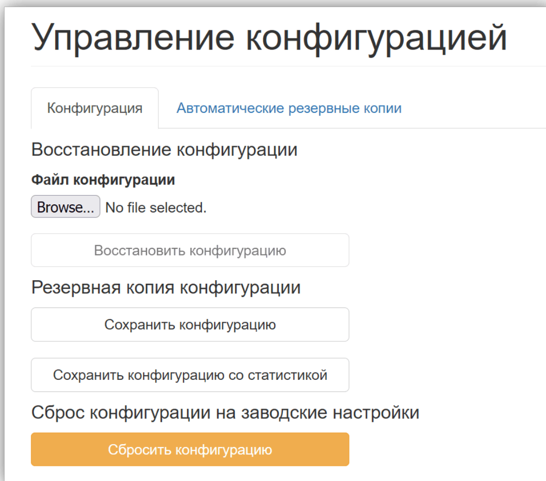
Рисунок 92. Вкладка конфигурации
