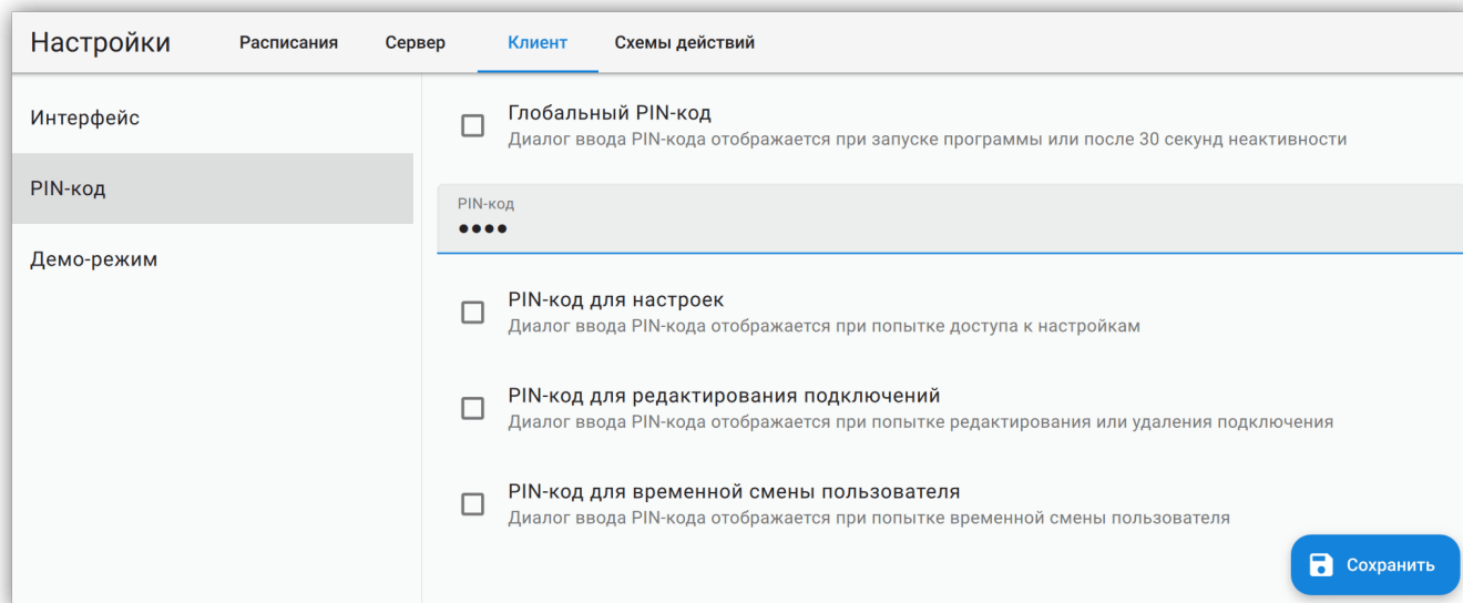
Рисунок 76. Настройки PIN-кода
