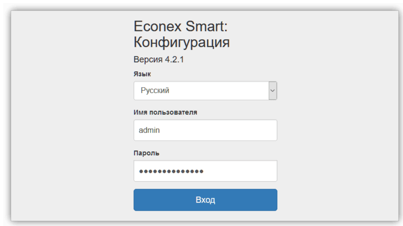
Рисунок 85. Страница авторизации
