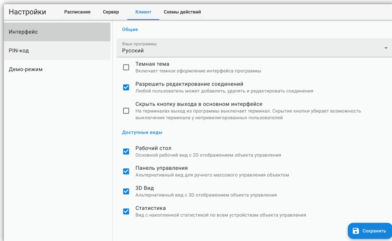
Рисунок 73. Настройки интерфейса
