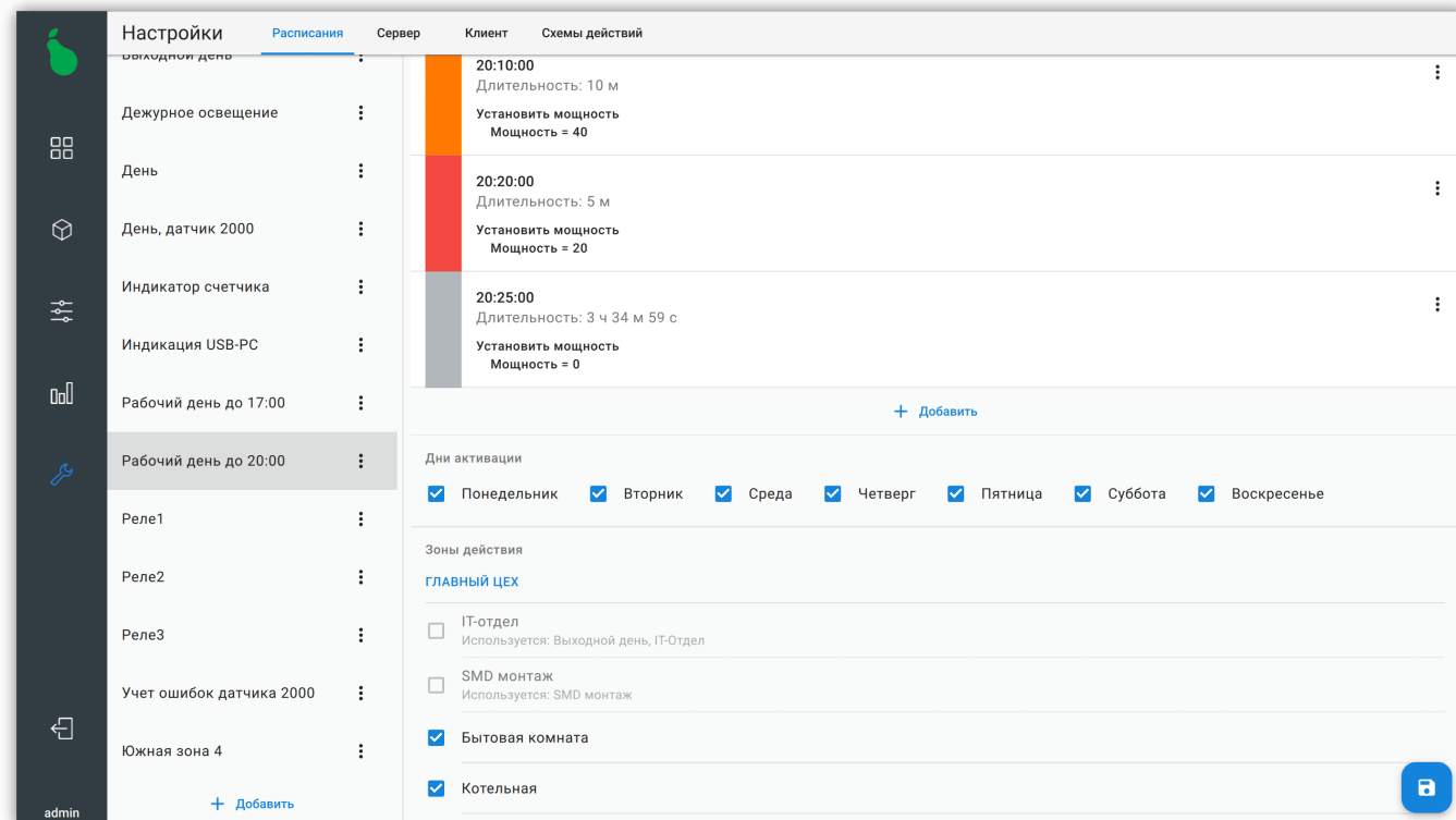
Рисунок 59. Редактирование расписаний
