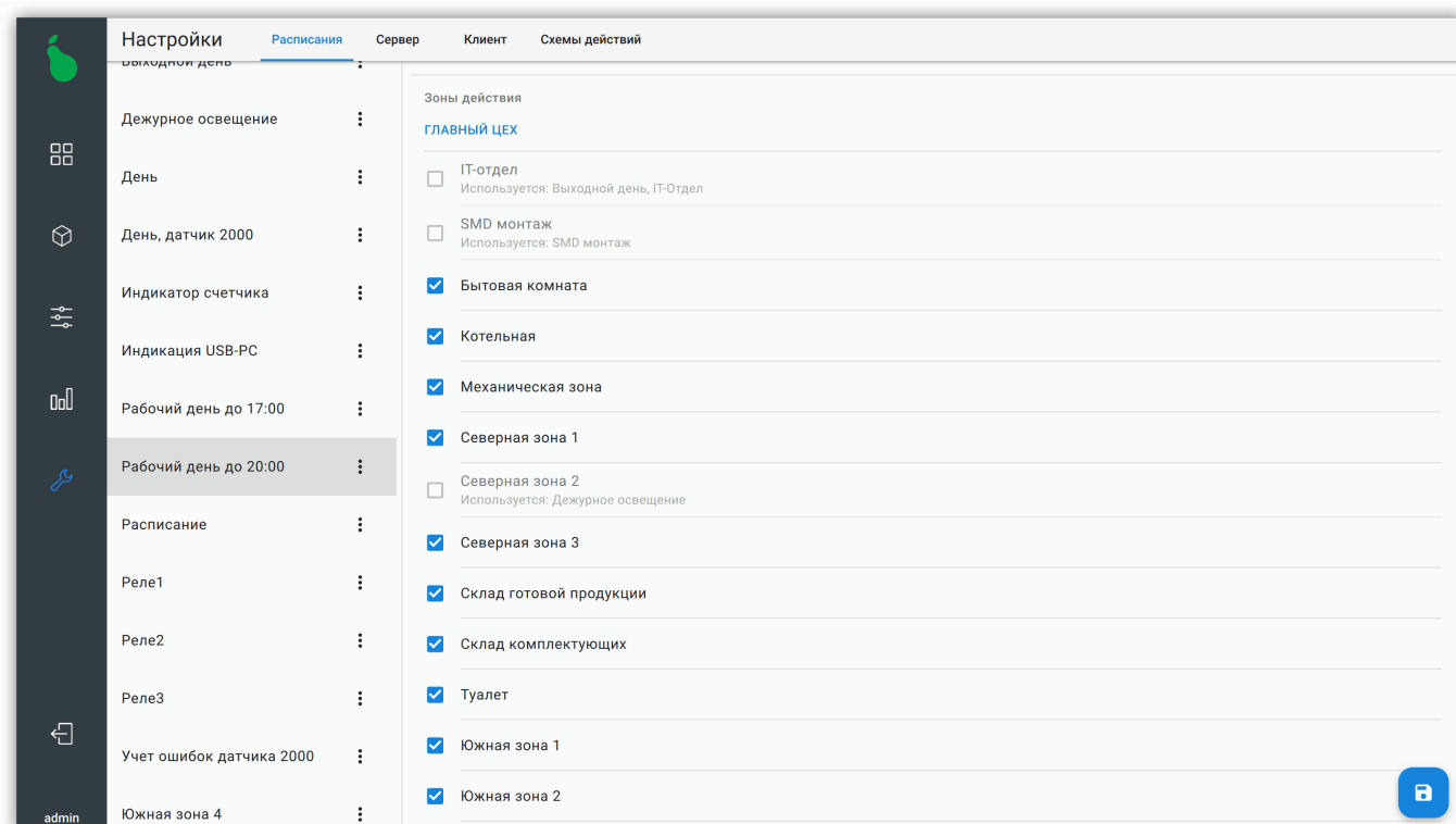
Рисунок 62. Зоны расписания
