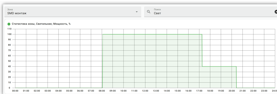
Рисунок 51. Сгруппированная статистика мощности светильников зоны
