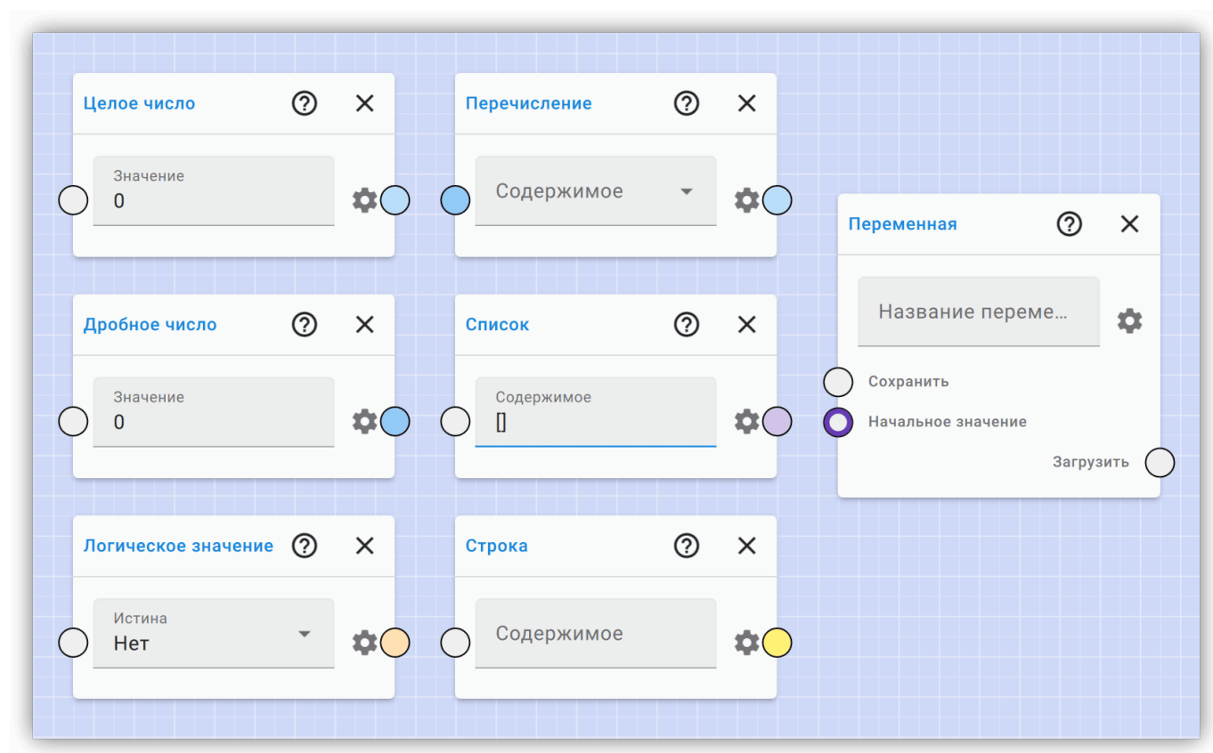
Рисунок 83. Входы и выходы различных типов данных
