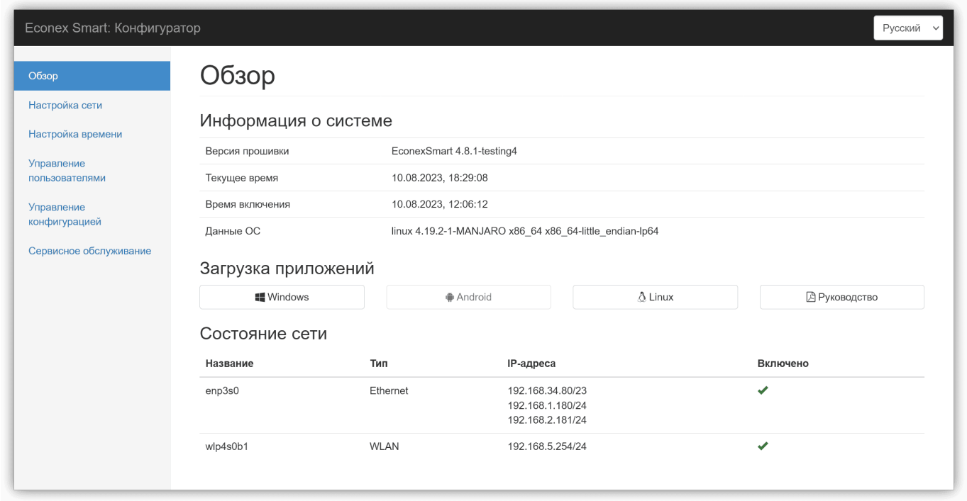
Рисунок 86. Общий вид веб-интерфейса, вкладка Обзор
