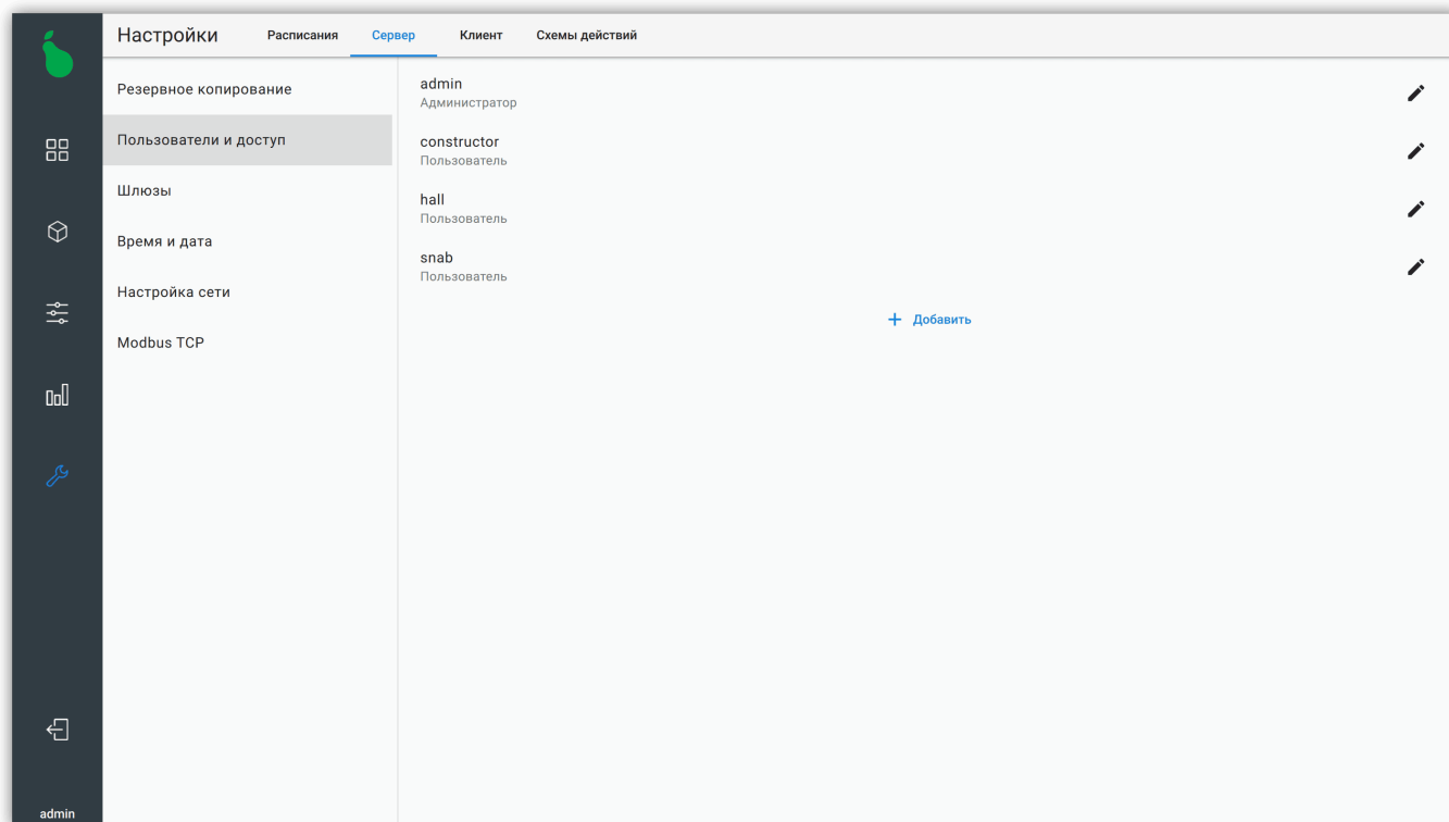
Рисунок 64. Список пользователей
