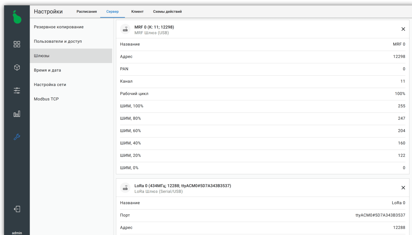
Рисунок 66. Настройка шлюзов
