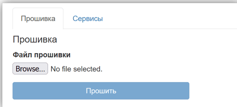
Рисунок 95. Вкладка "Прошивка"
