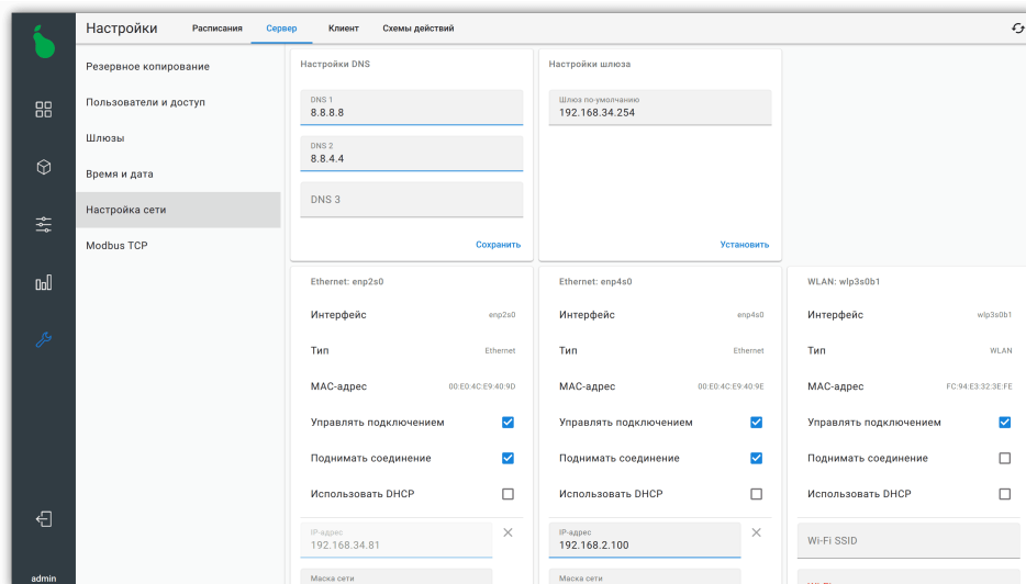
Рисунок 69. Настройки сети
