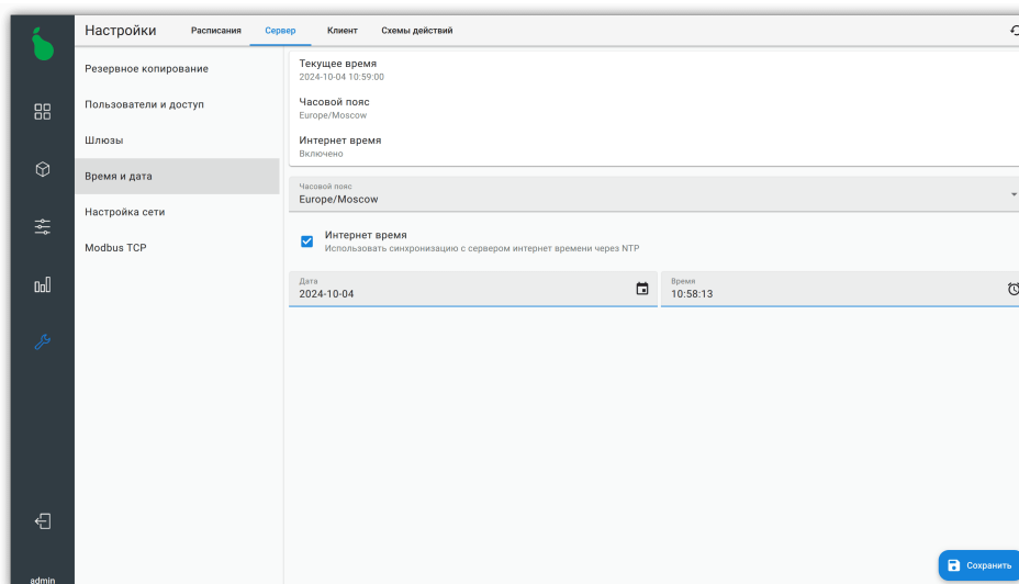
Рисунок 68. Настройки времени
