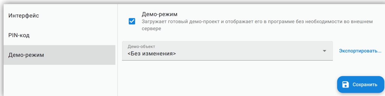
Рисунок 78. Настройки Демо-режима
