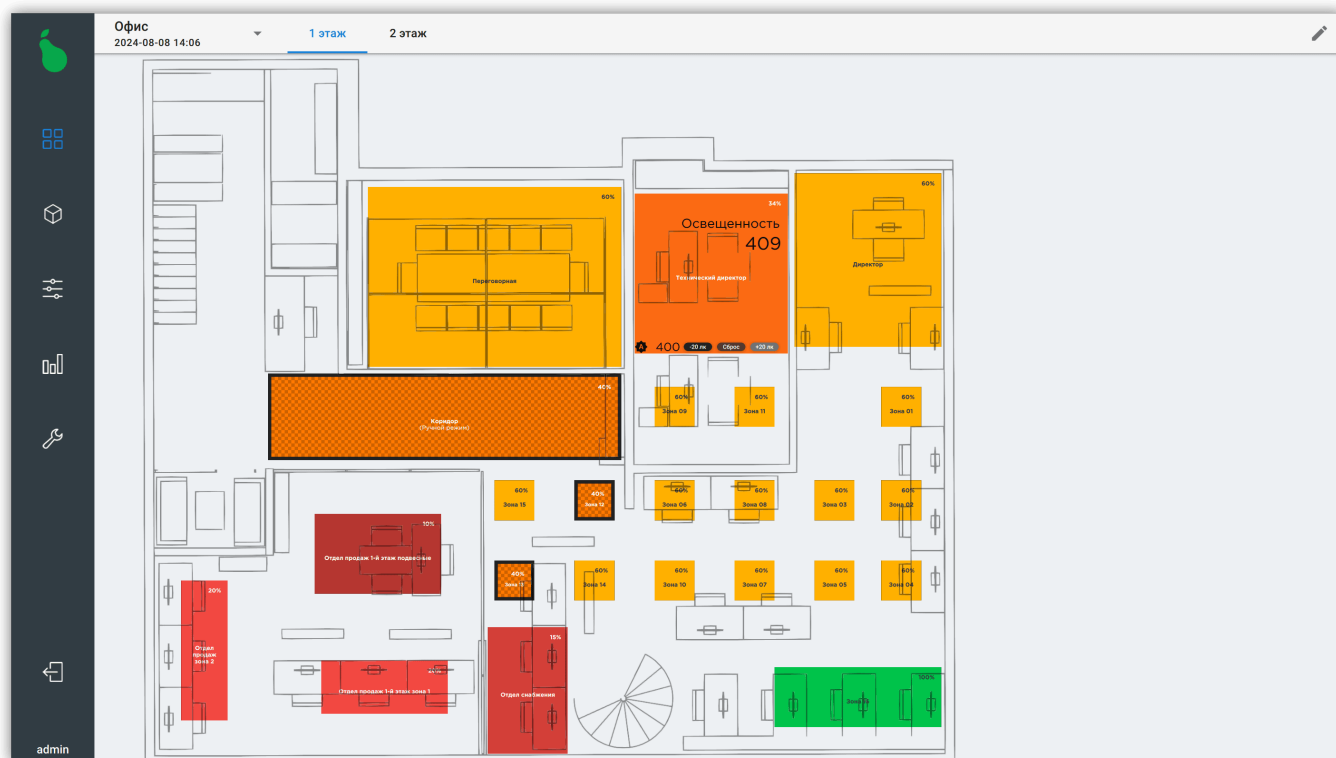
Рисунок 8. Рабочий стол
