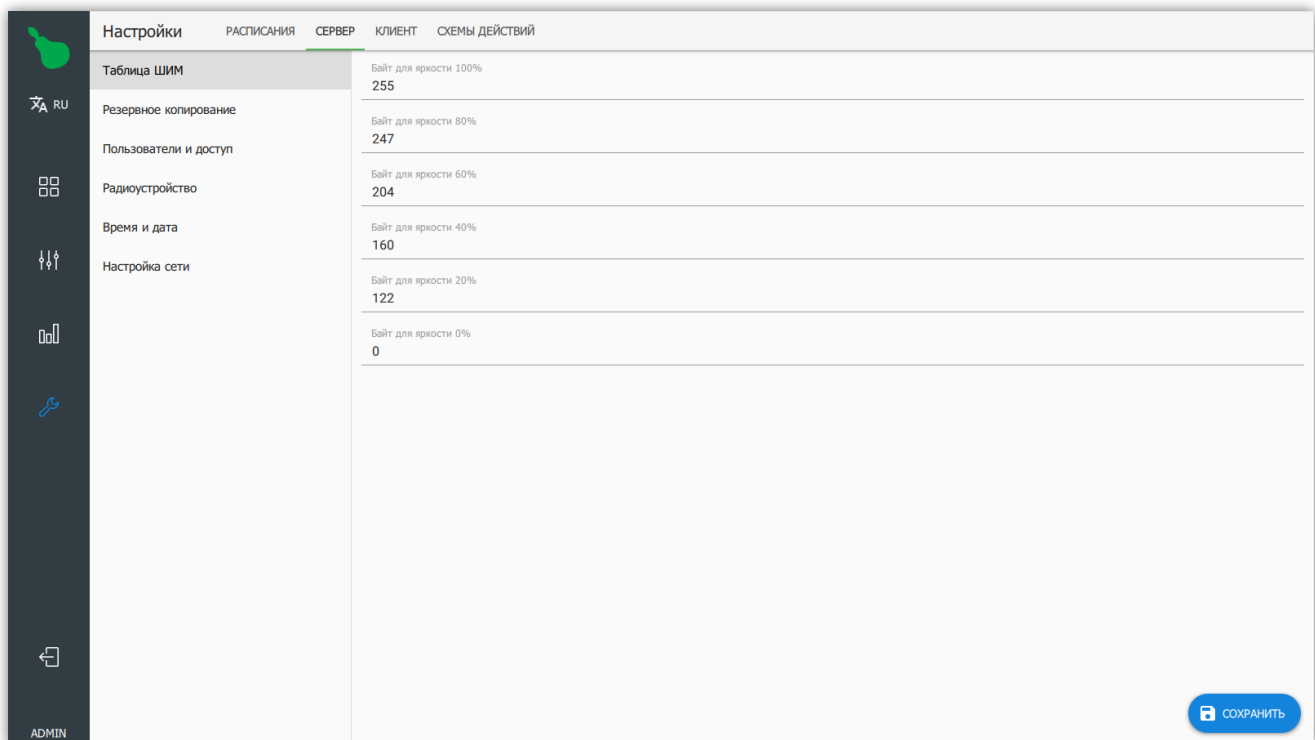
Рисунок 48. Настроенная таблица ШИМ для блоков питания Mean Well
