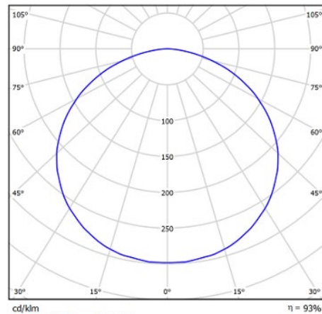
Рисунок 2. КСС типа Д (косинусная)
