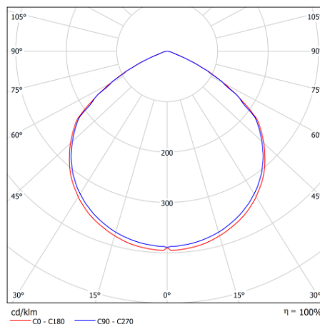
Рисунок 3. КСС типа Д120 (Косинусная)
