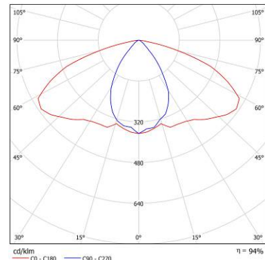
Рисунок 6. КСС типа Ш3 (Широкая осевая)
