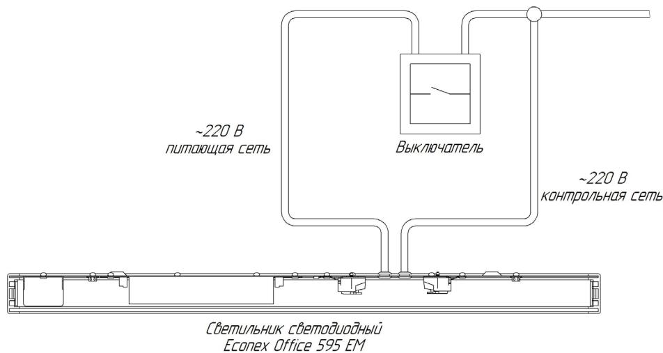
Рисунок 3. Схема подключение светильника серии Ecomex Office IP20 EM
