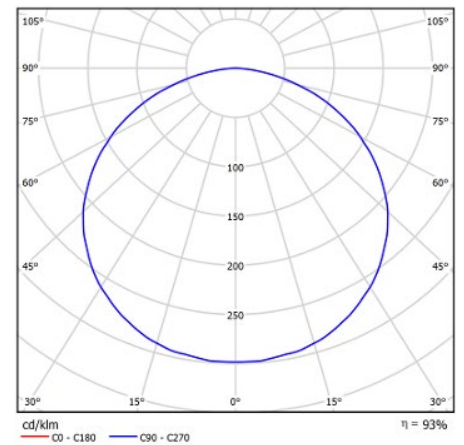
Рисунок 2. ККС типа Д (косинусная) ~220 В питающая сеть
