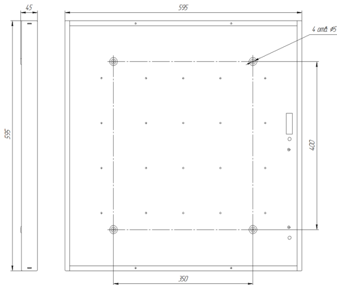
Рисунок 1. Габаритный чертеж Ecomex Office 595 EM
