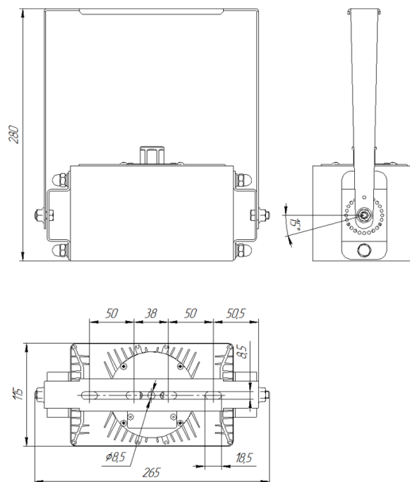
Рисунок 2 Габаритный чертеж светильника Econex PowerX Ex 20/30
