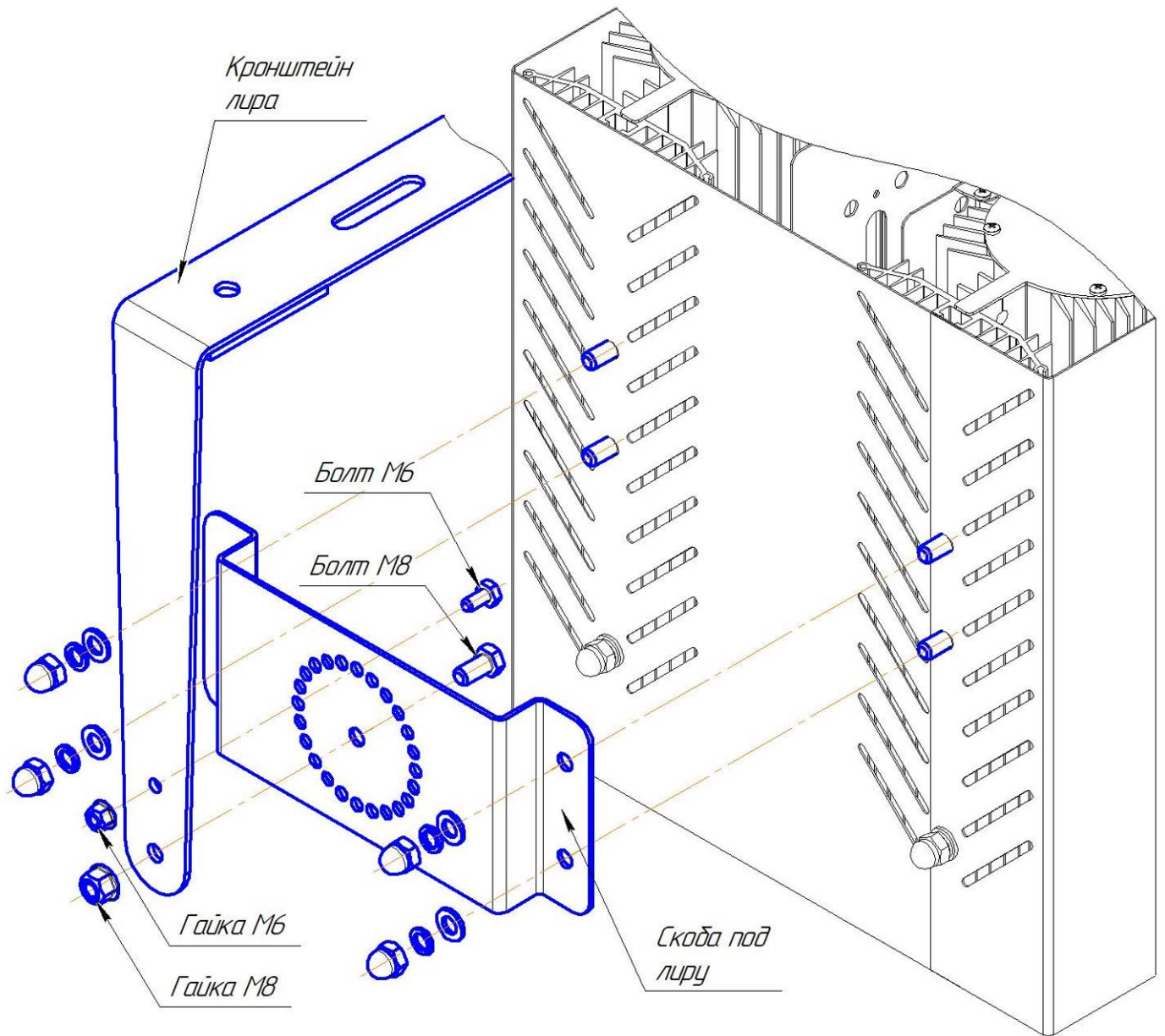
Рис.2 Установка комплекта.
