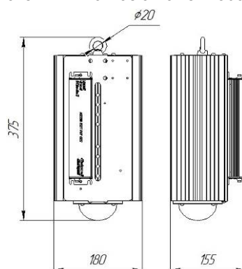
Рисунок 4. Габаритный чертеж Светильника Basic PowerX 120
