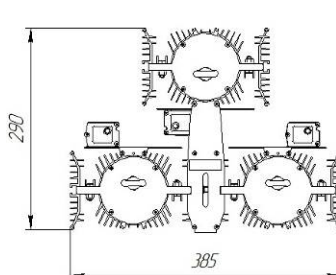
Рисунок 2. Габаритный чертеж светильника Basic PowerX 360
