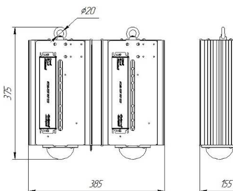
Рисунок 3. Габаритный чертеж светильника Basic PowerX 240
