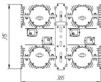
Рисунок 1. Габаритный чертеж светильника Basic PowerX 480
