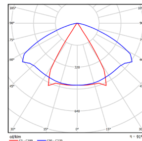
Рисунок 3. КСС типа Г60
