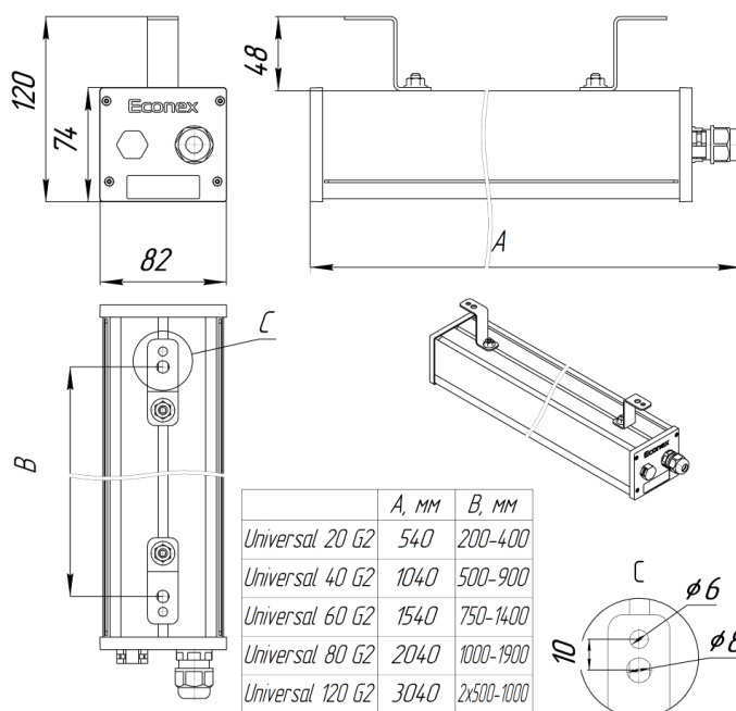
Рисунок 1. Габаритный чертеж светильника Econex Universal G2
