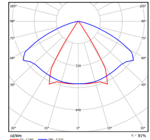
Рисунок 3. КСС типа G60
