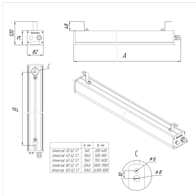
Рисунок 1. Габаритный чертеж светильника Ecomex Universal G2 ST
