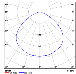
Рисунок 2. КСС типа D120
