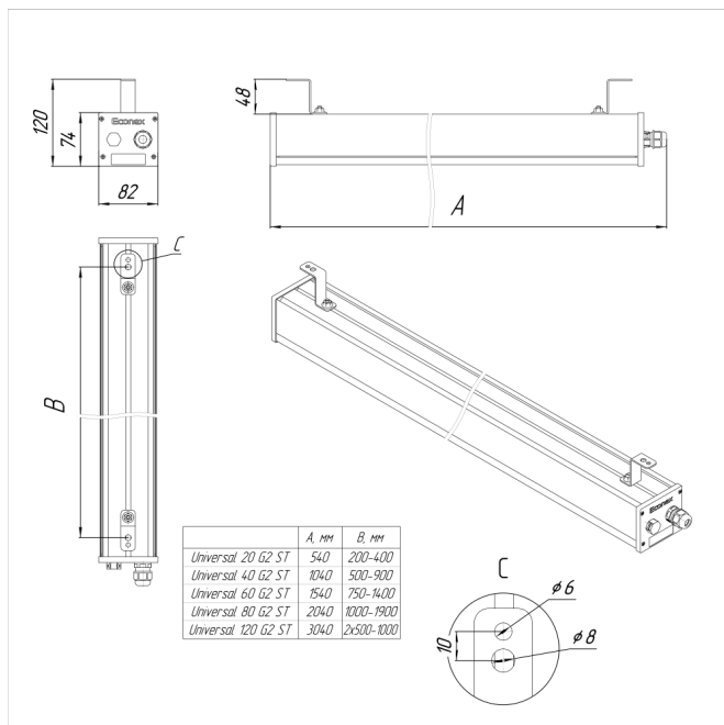
Рисунок 1. Габаритный чертеж светильника Econex Universal G2 ST
