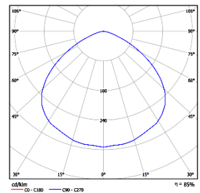
Рисунок 2. ККС типа Д120
