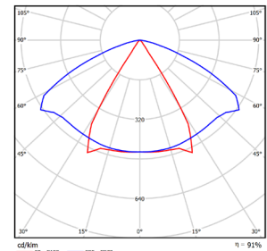
Рисунок 3. ККС типа Г60
