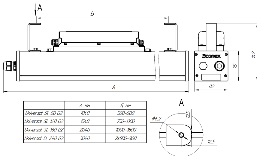
Рисунок 1. Габаритный чертеж светильника Ecomex Universal SL G2
