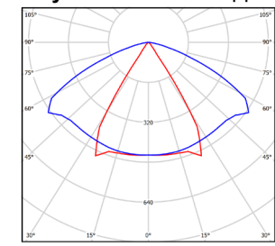
Рисунок 3. КСС типа Г60
