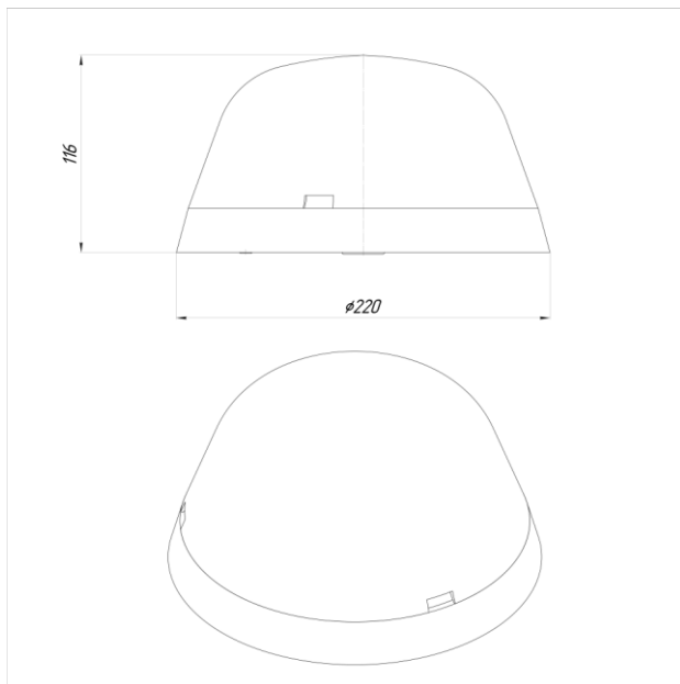
Рисунок 1. Габаритные размеры светильника Econex Budget 12/16 G3
