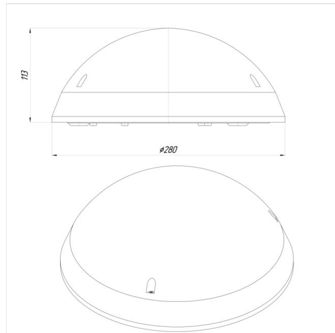
Рисунок 2. Габаритные размеры светильника Econex Budget 24/30 G3
