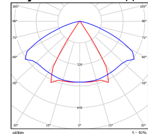
Рисунок 3. КСС типа Г60
