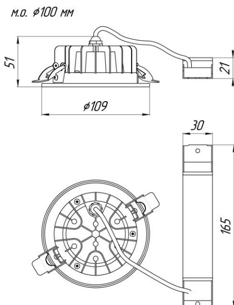
Рис. 1 - Габаритный чертеж Econex Downlight 12 G2
