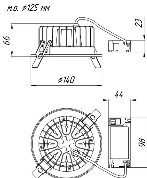
Рис. 2 - Габаритный чертеж Econex Downlight 15-20 G2
