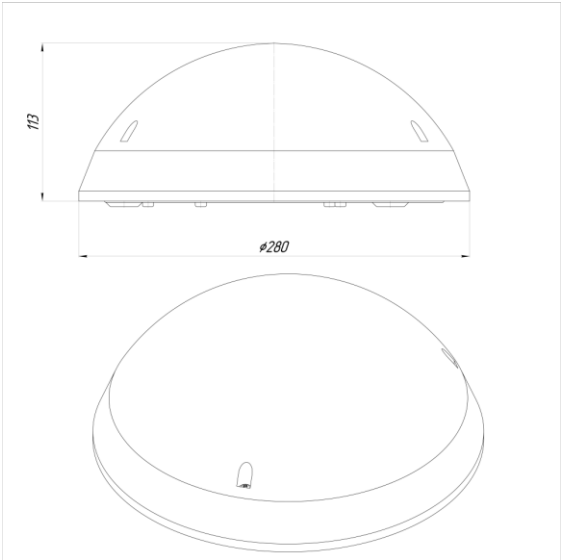
Рисунок 2. Габаритные размеры светильника Econex Budget 24/30 G3
