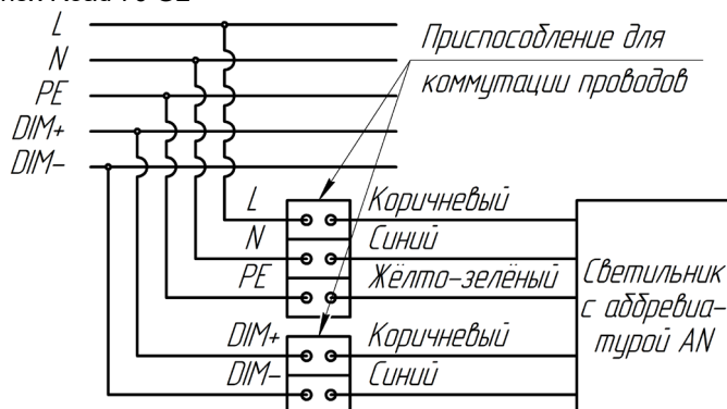
Рисунок 7. Схема электрическая для диммируемых светильников
