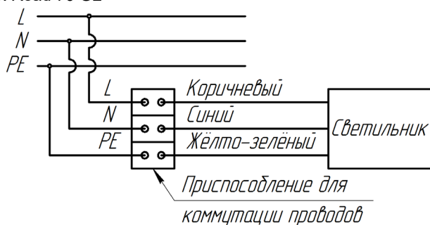
Рисунок 7. Схема электрическая
