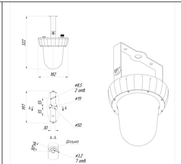
Рисунок 2. Габаритный чертеж светильника Ecomex Акорн Лира
