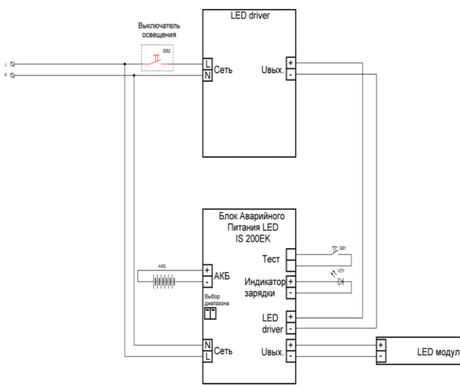
Рисунок 2. Схема подключение светильника Econex Office ES 690x370 EM
