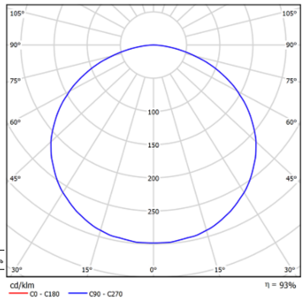
Рисунок 3. КСС типа Д (косинусная)
