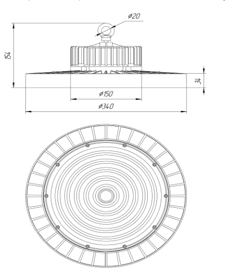
Рисунок 1. Габаритный чертеж светильника Econex Ray 60-100
