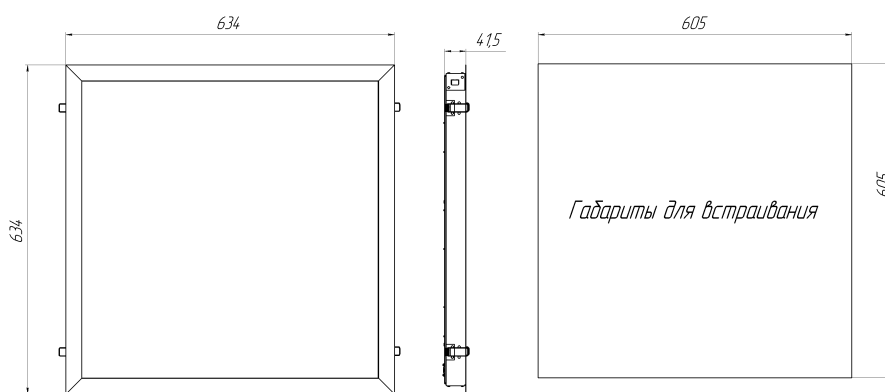
Рисунок 1. Габаритный чертеж Econex Office Gk 600x600 G2
