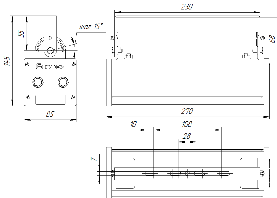
Рисунок 1. Габаритный чертёж светильника Ecomex Board G2
