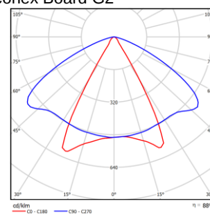
Рисунок 3. КСС типа G60
