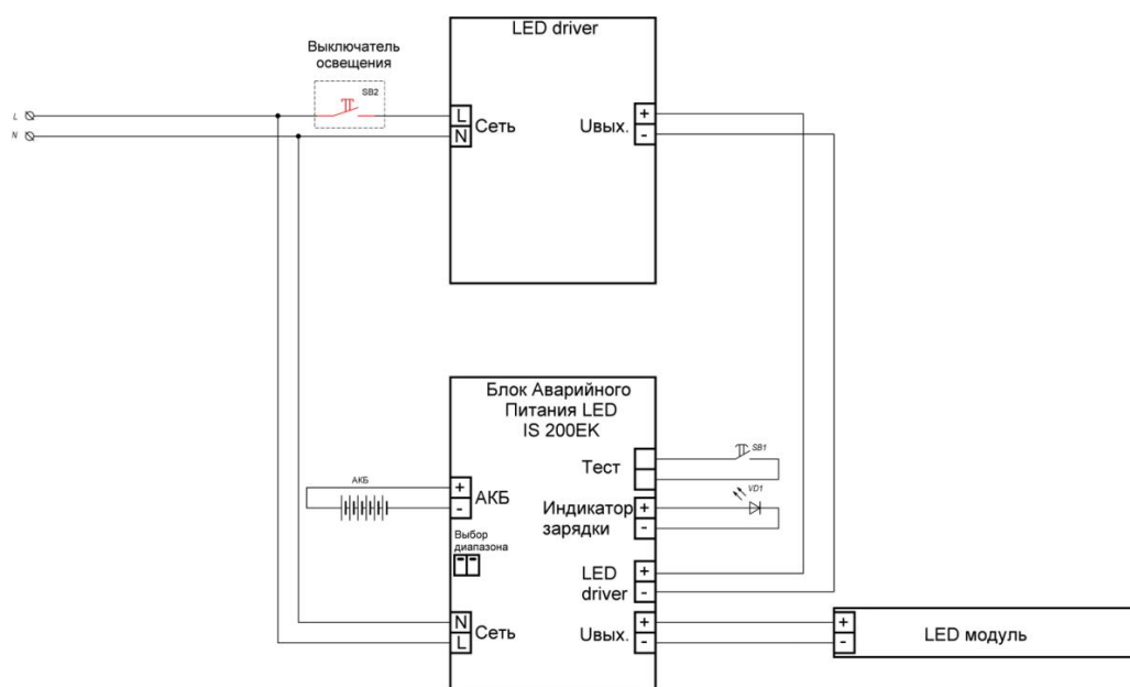
Рисунок 3. Схема электрическая
