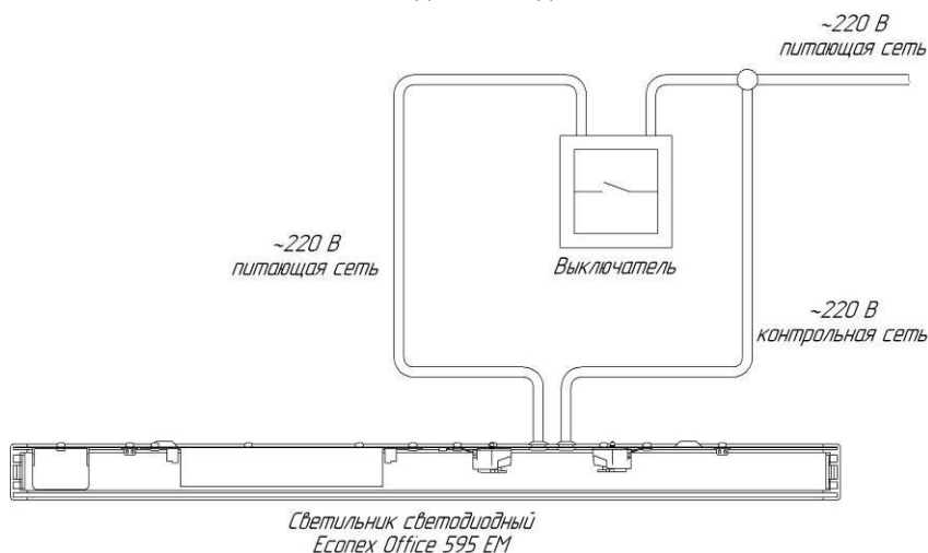
Рисунок 4. Схема подключения светильника серии Ecomex Office IP20 EM
