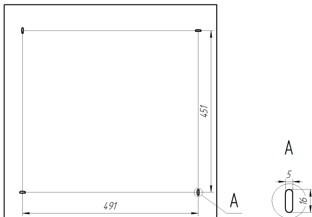
Рисунок 2. Расположение установочных отверстий на корпусе светильника Ecomex Office 595 для накладного монтажа.
