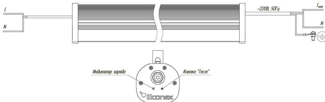
Рисунок 4. Подключение светодиодного светильника Ecomex Loft EM
