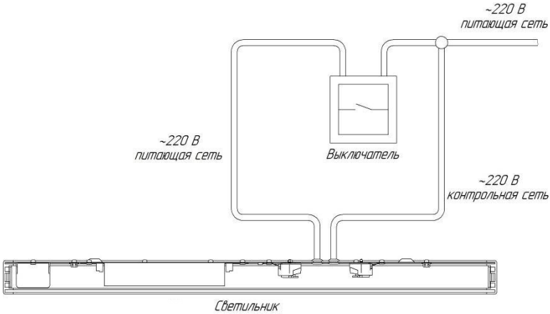
Рисунок 3. Схема подключение светильника Gr 1215x312 G2 EM
