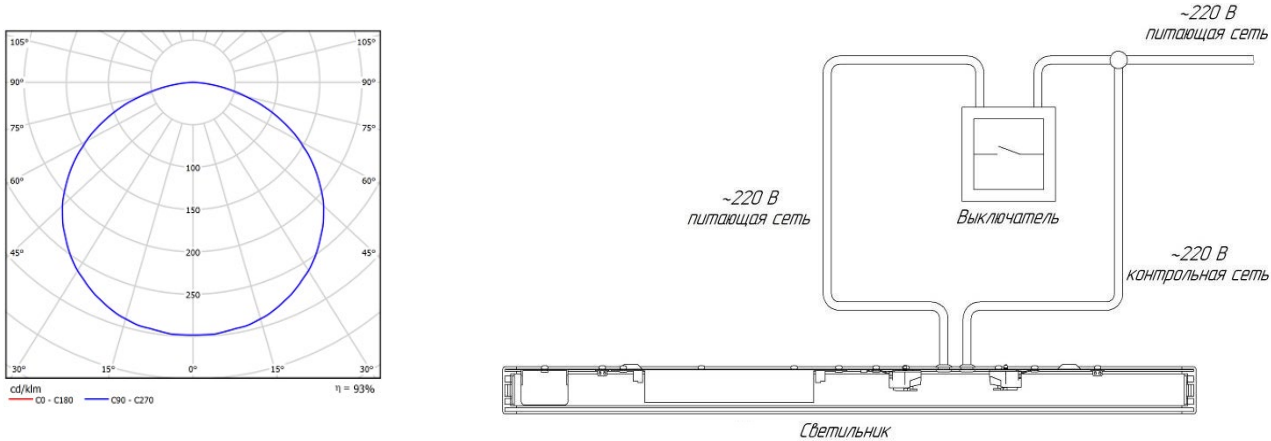
Рисунок 2. КСС типа «Косинусная»
