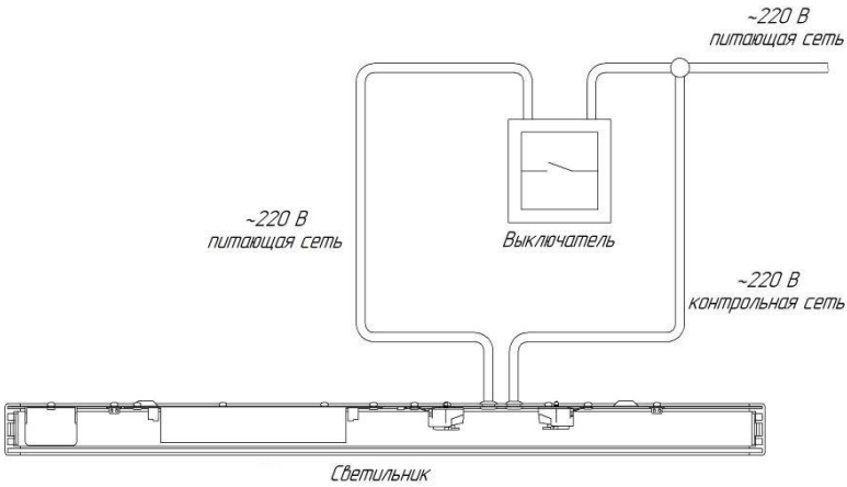
Рисунок 3. Схема подключение светильника Gr 1188x288 G2 EM
