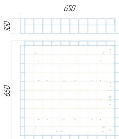
Рисунок 1. Габаритный чертеж Econex Office S 650x650 G2
