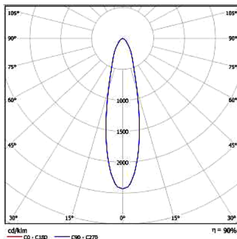
Рисунок 1. КСС типа K15 (Концентрированная)
