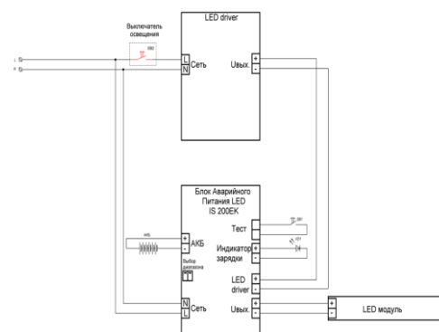
Рисунок 3. Схема подключения светильника Ecomex Office EGk 600x600 EM
