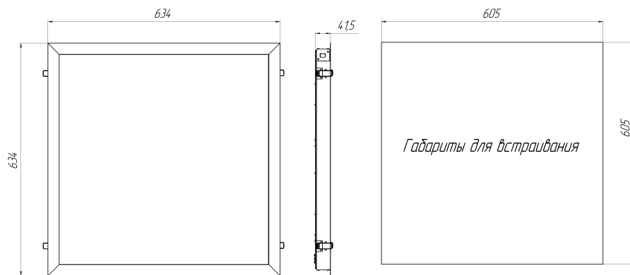
Рисунок 1. Габаритный чертеж Ecomex Office EGk 600x600
