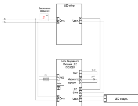
Рисунок 3. Схема подключение светильника Ecomex Office EGr 1215x312 EM
