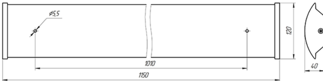
Рисунок 1. Габаритный чертеж Ecomex Office 1200 AN
