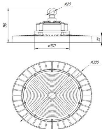
Рисунок 1. Габаритный чертеж светильника Ecomex Ray 100 и 150
