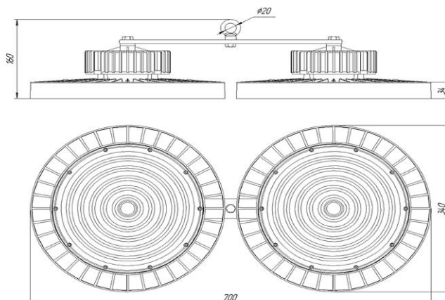
Рисунок 4. Габаритный чертеж светильника Ecomex Ray 400
