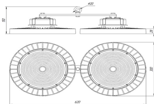
Рисунок 3. Габаритный чертеж светильника Ecomex Ray 300
