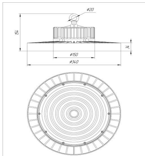
Рисунок 2. Габаритный чертеж светильника Ecomex Ray 200
