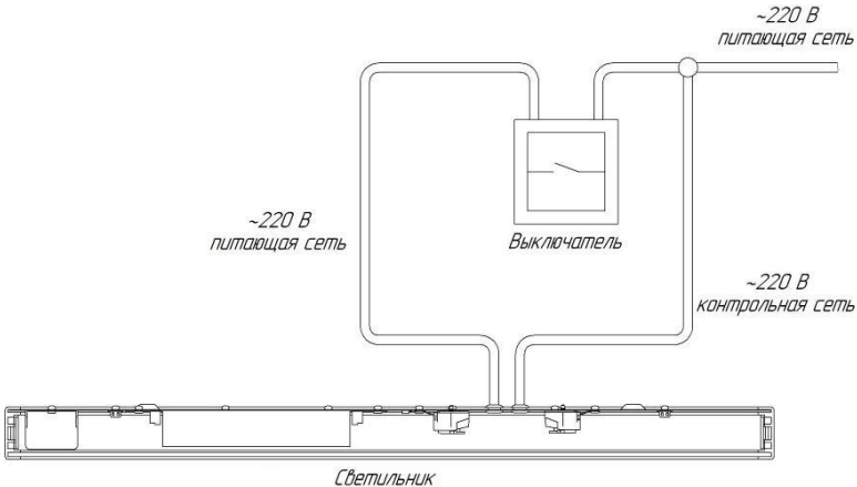
Рисунок 3. Схема подклчение светильника Gr 588x588 G2 EM
